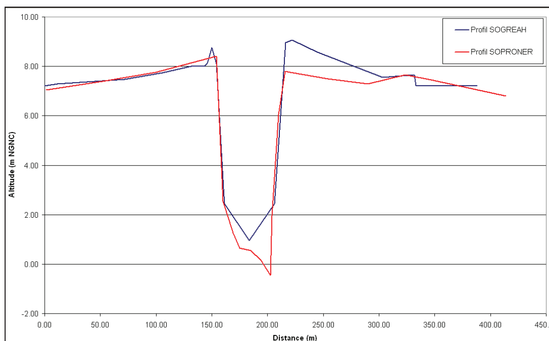
Comparaison des profils SOGREAH et SOPRONER en amont du pont de la RT1
