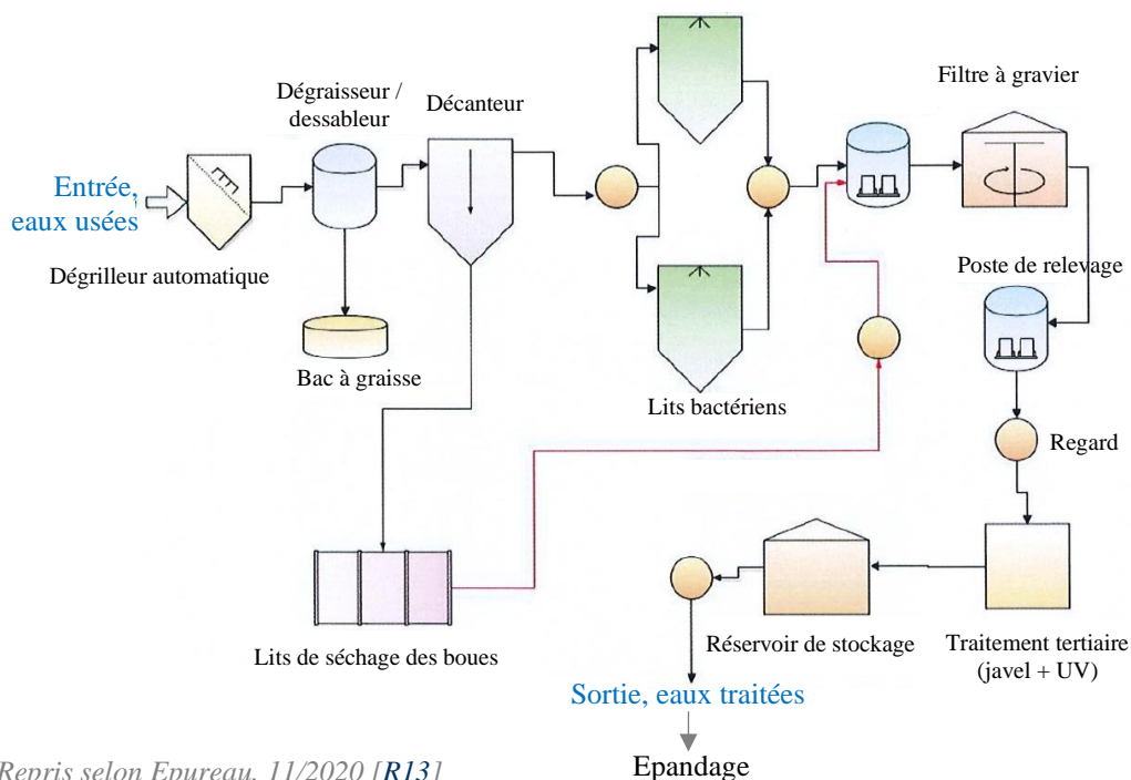
Figure 02 : Synoptique simplifié de la filière de traitement
