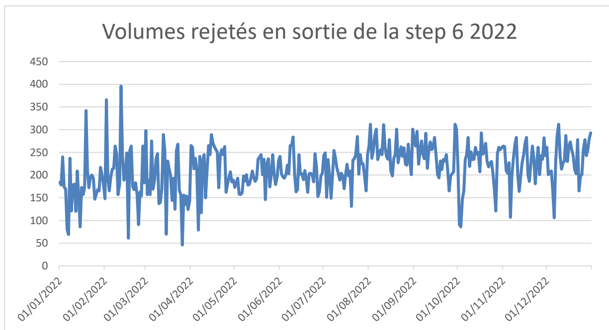
Figure 2 : Volumes journaliers de rejet en sortie de la STEP 6 en 2022
