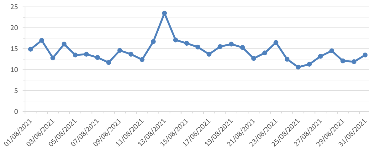
Mesure de turbidité (en NTU) en continu - Rejets effluents industriels (6-IP1)
