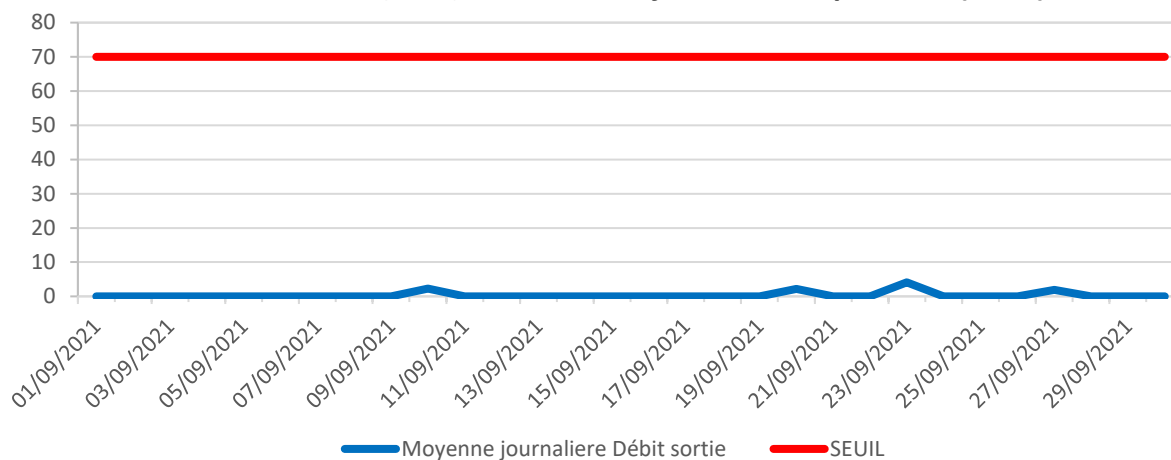
Mesure de débit (m 3 /h) en continu - Rejets effluents pluviaux (6-IP2)
