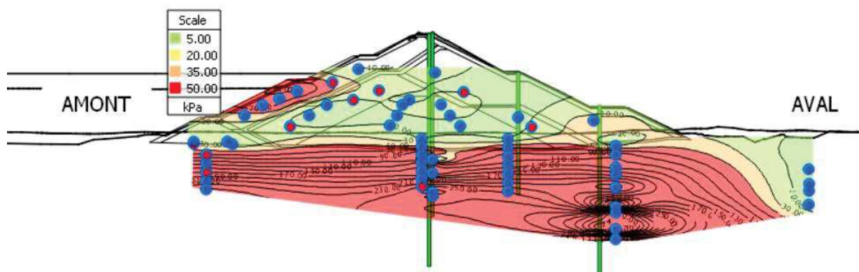
Figure 8 : Isoligne de pression interstitielle en kPa – Chainage 700 en date du 30/04/2025
