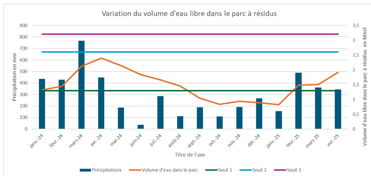
Figure 2 : Variation du volume d'eau par rapport aux valeurs seuils du TARP
