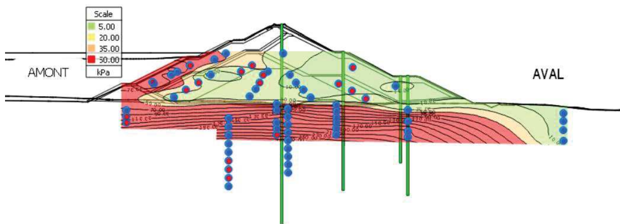
Figure 7 : Isoligne de pression interstitielle en kPa – Chainage 500 en date du 30/04/2025
