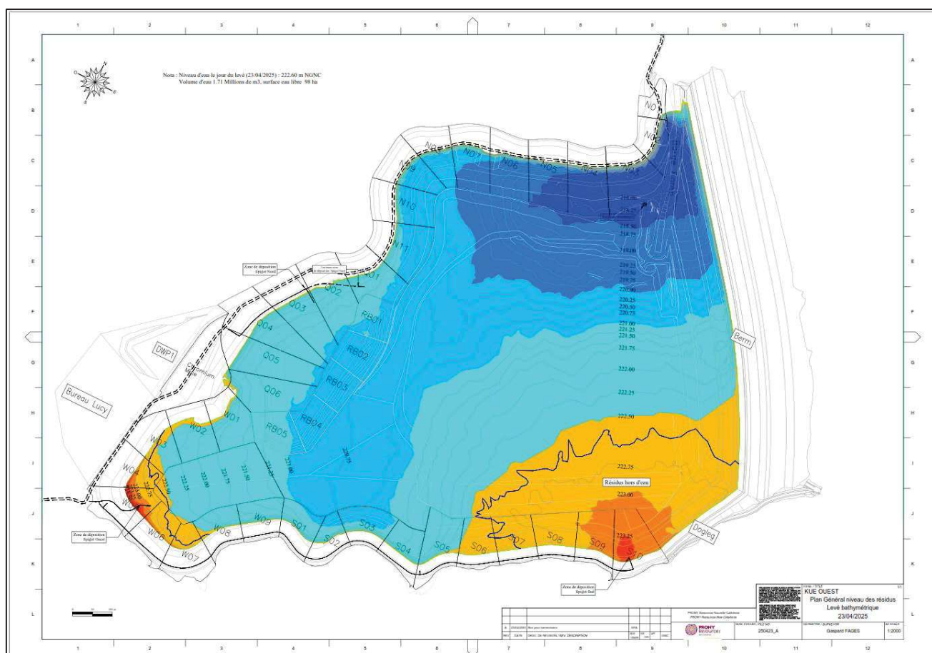
Figure 1 : Plage de déposition selon le levé bathymétrique du 23 avril 2025
