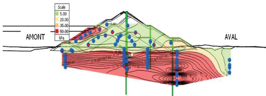
Figure 6 : Isoline de pression interstitielle en kPa – Chainage 700 en date du 31/05/2025
