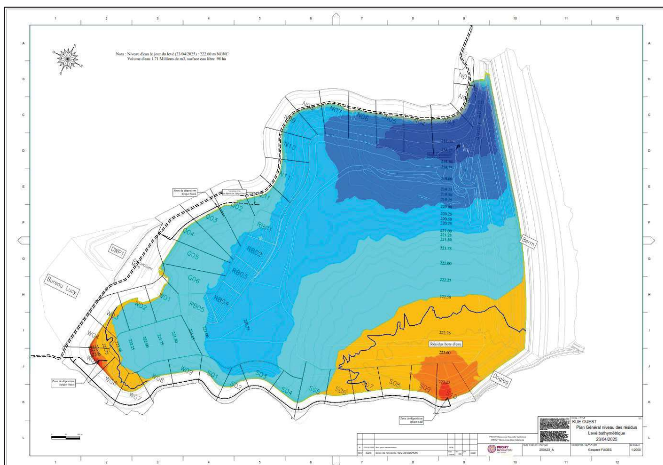
Figure 1 : Plage de dépôt selon le levé bathymétrique du 23 avril 2025
