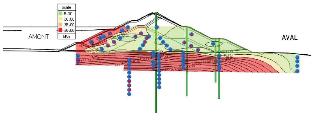
Figure 5 : Isoligne de pression interstitielle en kPa – Chainage 500 en date du 31/05/2025
