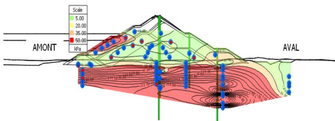
Figure 6 : Isoligne de pression interstitielle en kPa – Chainage 700 en date du 30/06/2025
