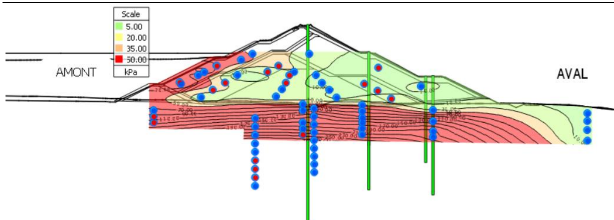
Figure 5 : Isoligne de pression interstitielle en kPa – Chainage 500 en date du 30/06/2025
