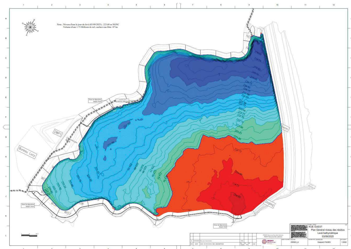
Figure 1 : Plage de déposition selon le levé bathymétrique du 3 septembre 2025
