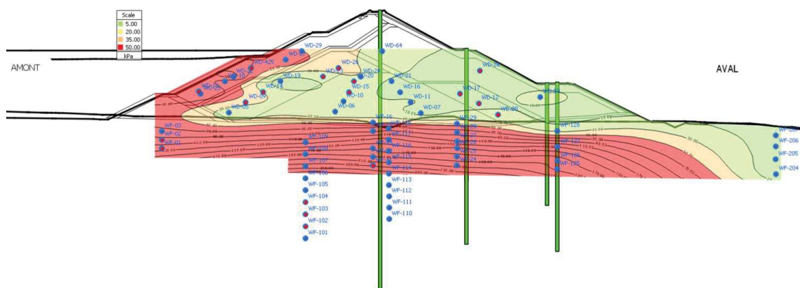
Figure 8 : Isoligne de pression interstitielle en kPa – Chainage 500 en date du 30/09/2025
