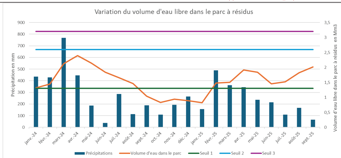
Figure 5 : Variation du volume d'eau par rapport aux valeurs seuils du TARP
