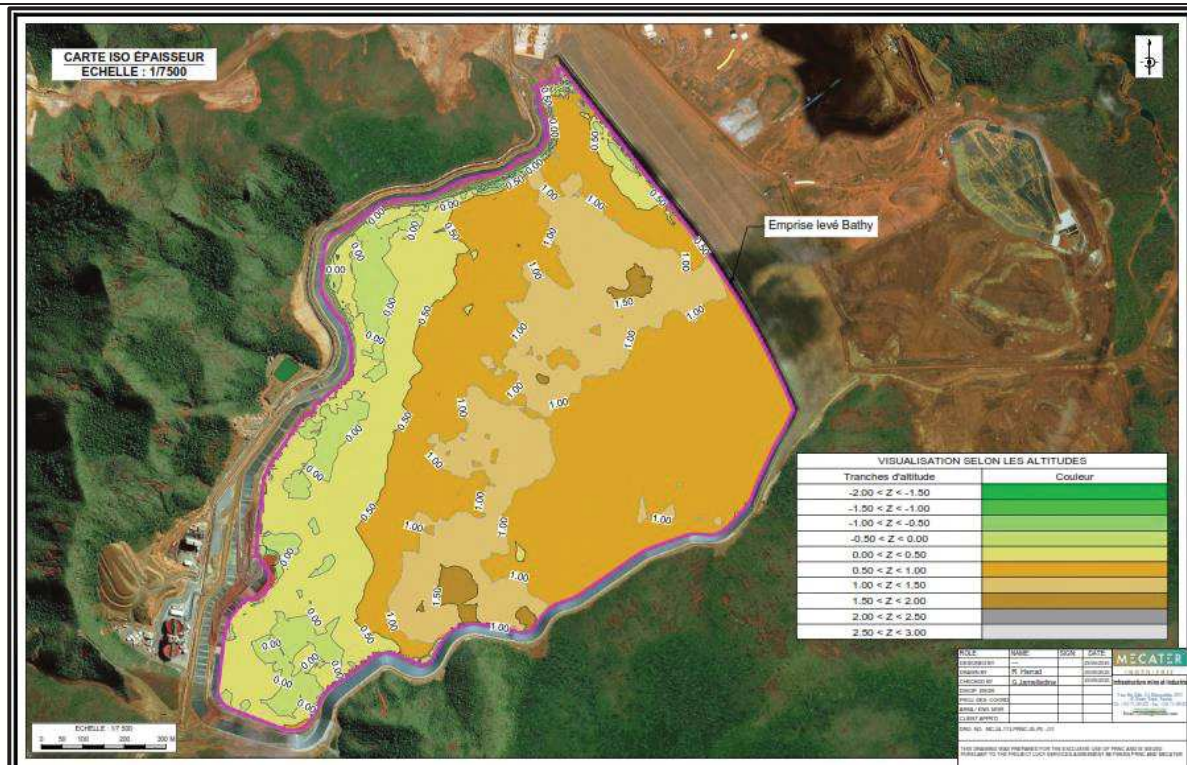
Figure 4 : Plan de déposition des résidus entre juin et septembre 2025 - Carte d'iso-épaisseur des résidus déposés pendant cette période
