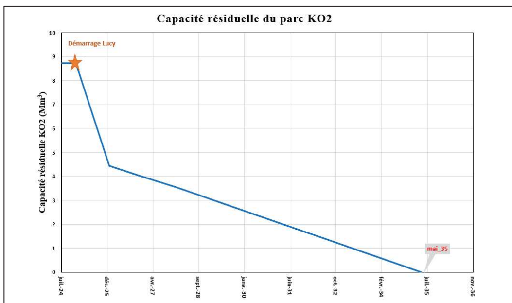
Figure 7 : Graphique - capacité résiduelle dans KO2 avec projet Lucy
