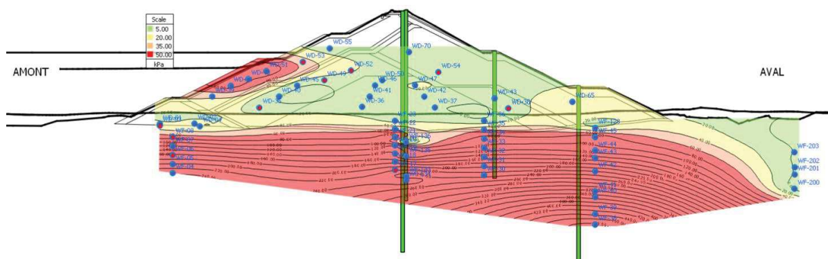
Figure 9 : Isoligne de pression interstitielle en kPa – Chainage 700 en date du 30/09/2025
