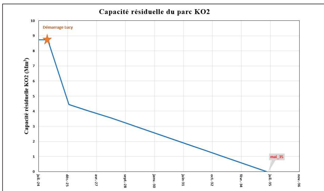
Figure 6 : Graphique - capacité résiduelle dans KO2 avec projet Lucy
