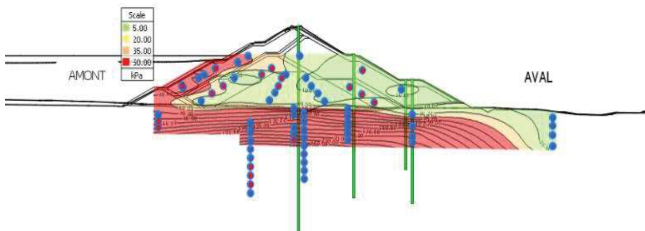
Figure 7 : Isoligne de pression interstitielle en kPa – Chainage 500 en date du 31/08/2025
