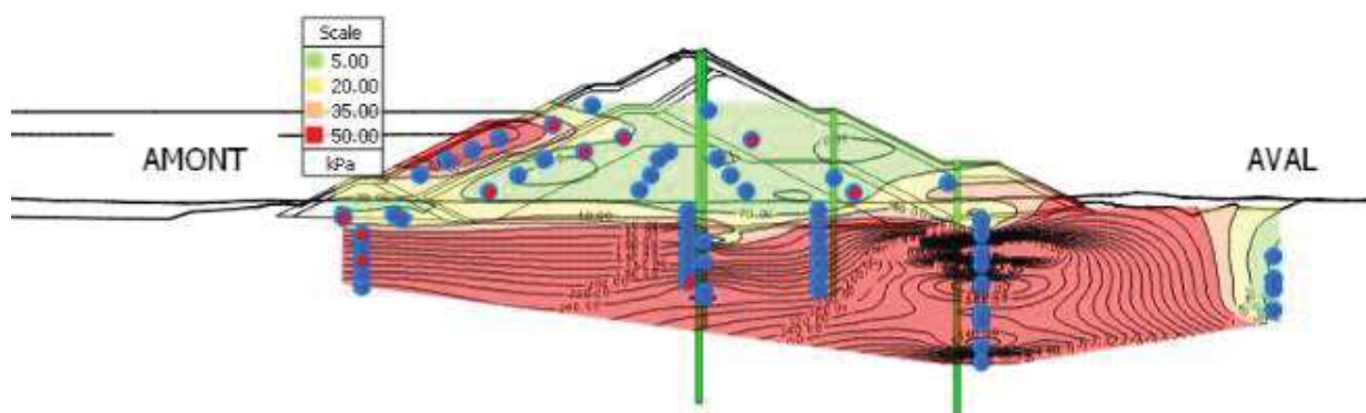
Figure 8 : Isoligne de pression interstitielle en kPa – Chainage 700 en date du 31/08/2025
