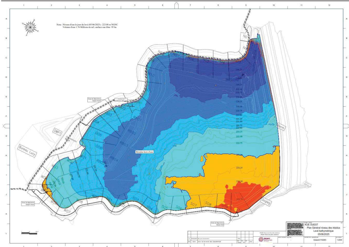
Figure 1 : Plage de déposition selon le levé bathymétrique du 5 juin 2025
