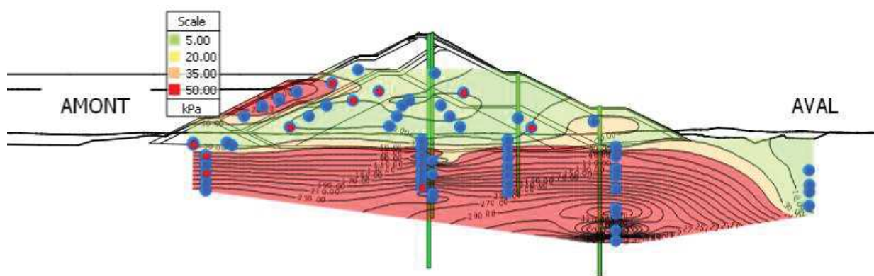
Figure 8 : Isoligne de pression interstitielle en kPa – Chainage 700 en date du 31/07/2025
