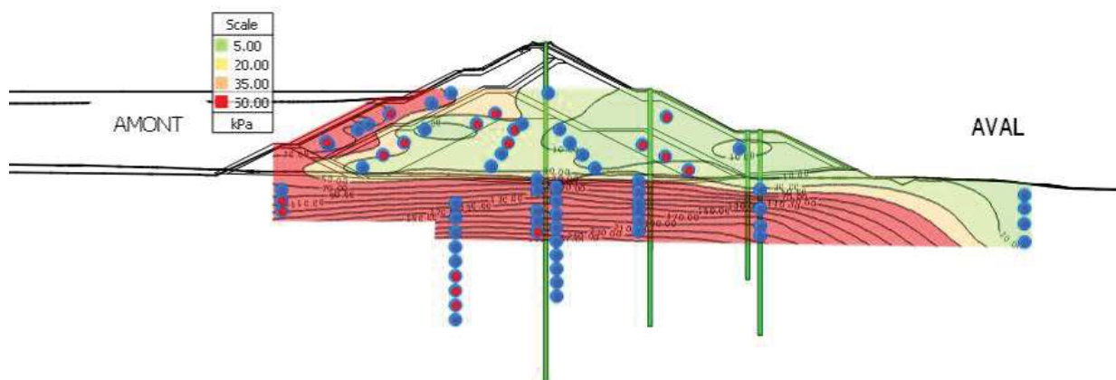
Figure 7 : Isoligne de pression interstitielle en kPa – Chainage 500 en date du 31/07/2025
