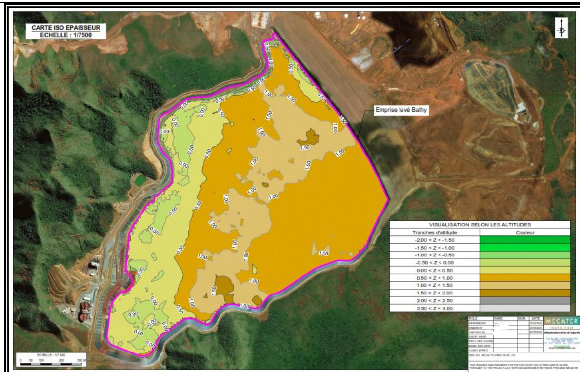
Figure 4 : Plan de dépôt des résidus entre juin et septembre 2025 - Carte d'iso-épaisseur des résidus déposés pendant cette période
