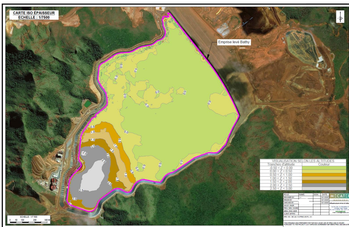
Figure 5 : Plan de dépôt des résidus entre septembre 2025 et octobre 2025 - Carte d'iso-épaisseur des résidus déposés pendant cette période
