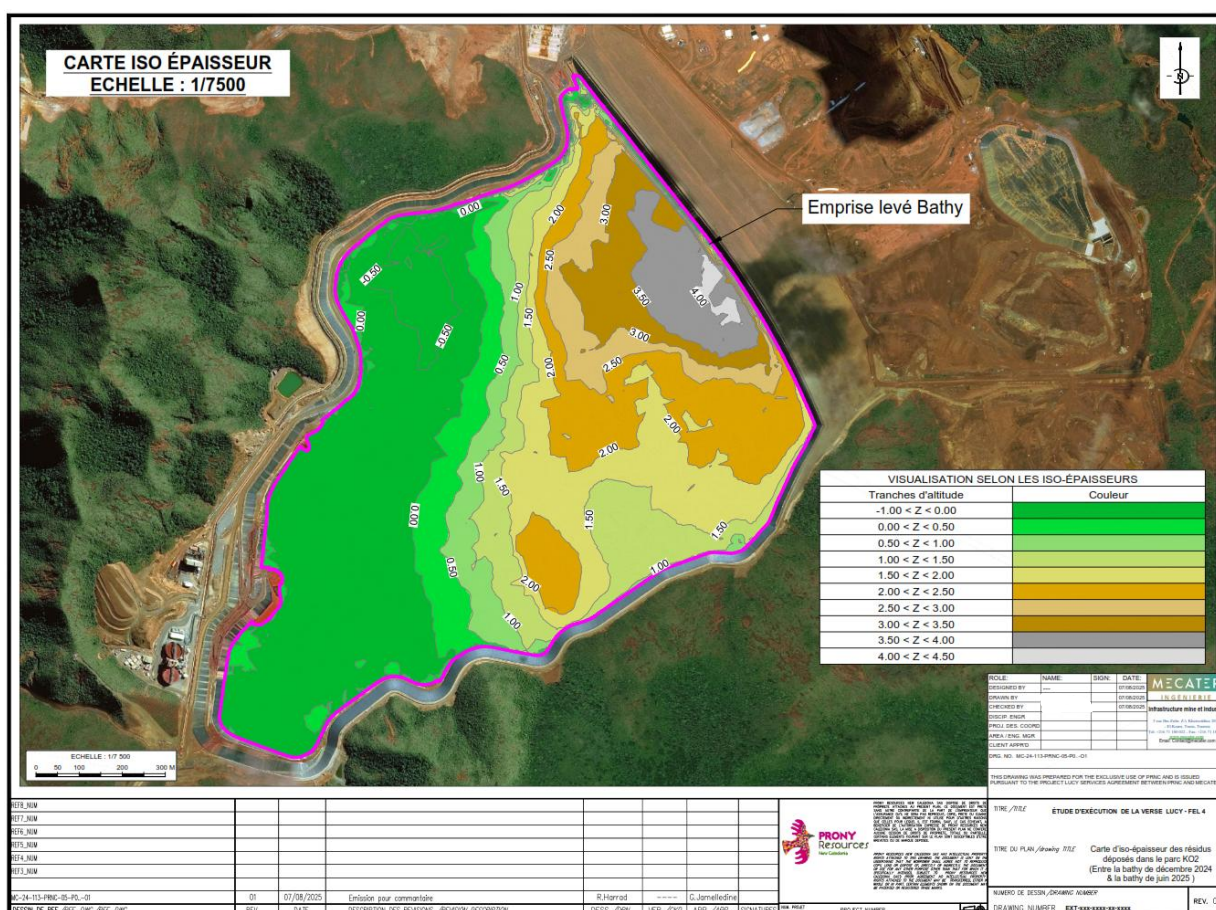
Figure 3 : Plan de déposition des résidus entre décembre 2024 et juin 2025 - Carte d'iso-épaisseur des résidus déposés pendant cette période
