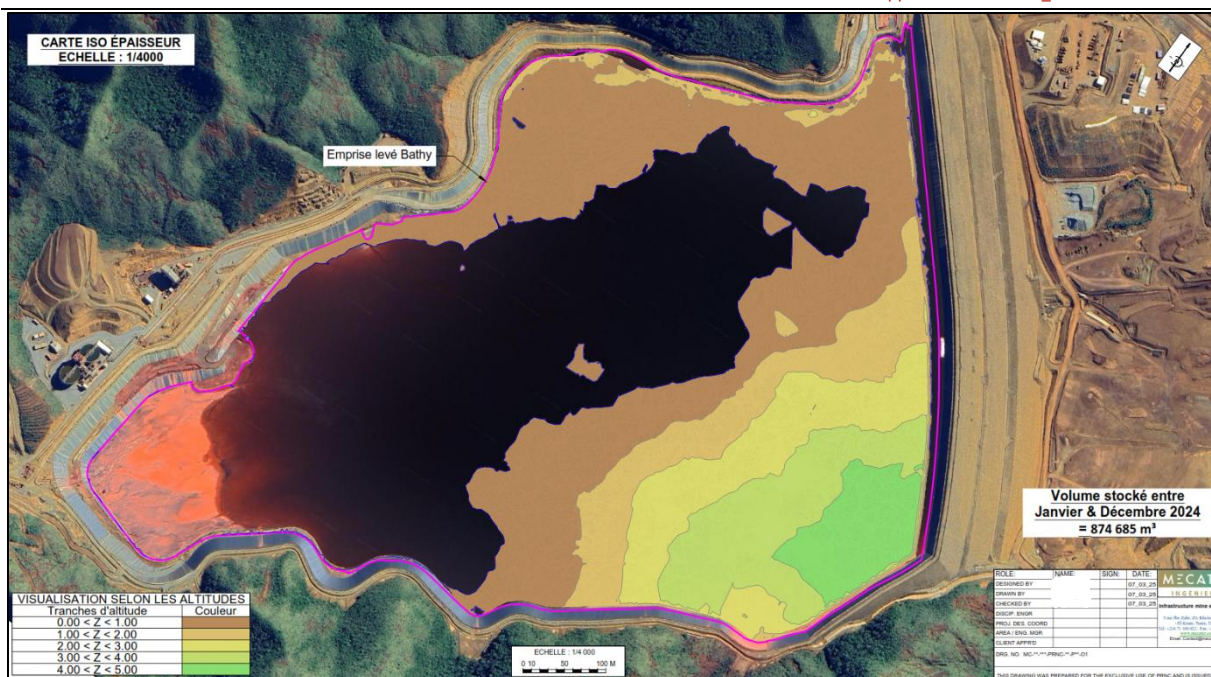
Figure 2 : Plan de déposition des résidus entre janvier et décembre 2024 – Carte d’iso-épaisseur de résidus déposés pendant cette période
