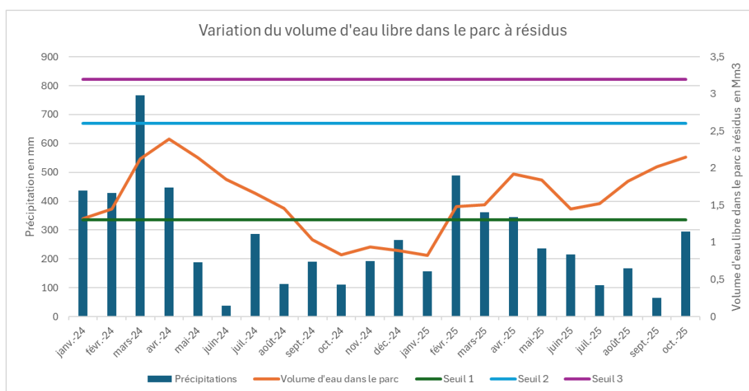
Figure 6 : Variation du volume d'eau par rapport aux valeurs seuils du TARP
