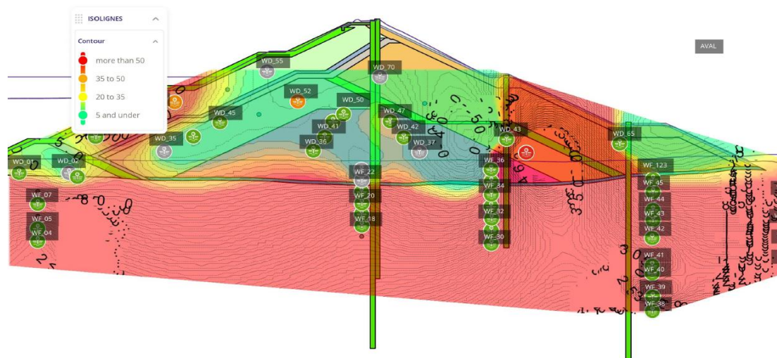
Figure 10 : Isoligne de pression interstitielle en kPa – Chainage 700 en date du 30/11/2025
