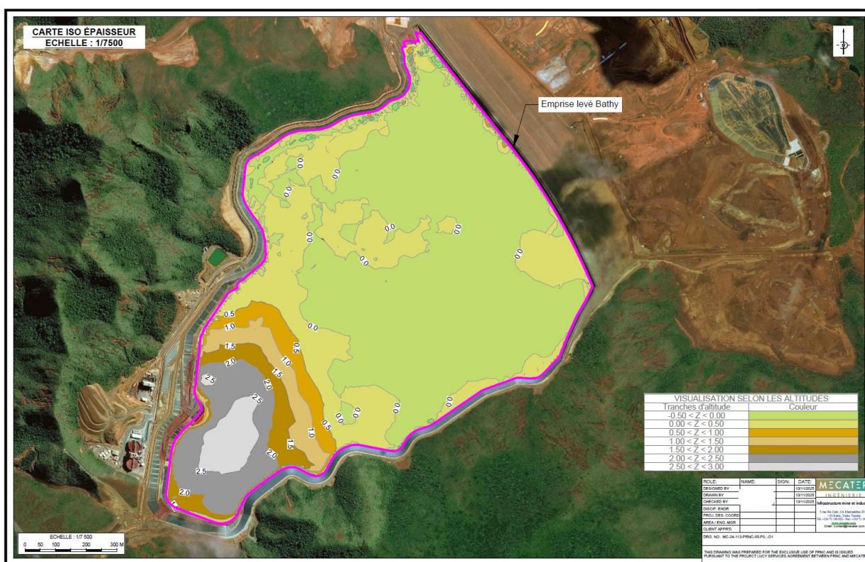
Figure 5 : Plan de déposition des résidus entre septembre 2025 et octobre 2025 - Carte d'iso-épaisseur des résidus déposés pendant cette période
