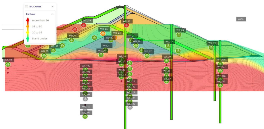
Figure 9 : Isoligne de pression interstitielle en kPa – Chainage 500 en date du 30/11/2025
