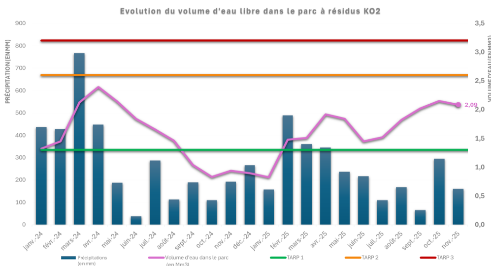
Figure 6 : Variation du volume d'eau par rapport aux valeurs seuils du TARP
