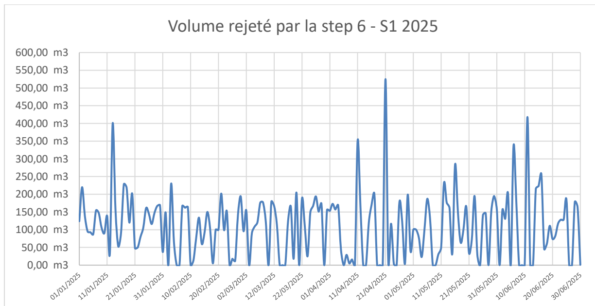
Figure 2 : Volumes journaliers de rejet en sortie de la STEP 6 en 2025
