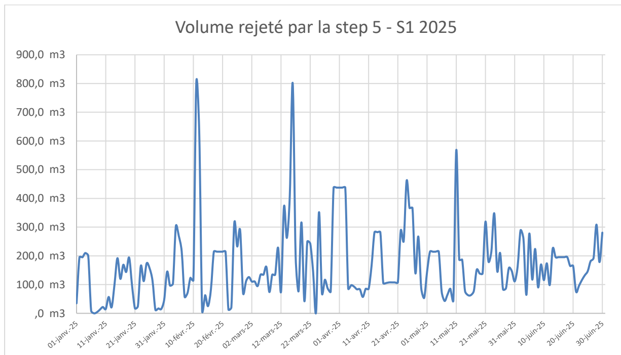
Figure 1 : Débits journaliers de rejet en sortie de la STEP 5 - 2025
