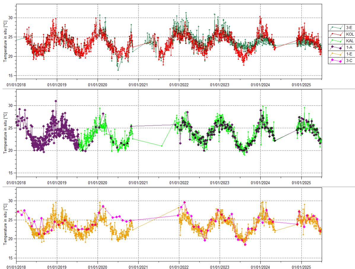
Figure 31 : Données de températures prises à fréquence journalière aux stations 3-E, KOL, KAL, 1-E, à fréquence hebdomadaire à 1-A et à fréquence mensuelle à 3-C entre janvier 2018 et le 1er juillet 2025
