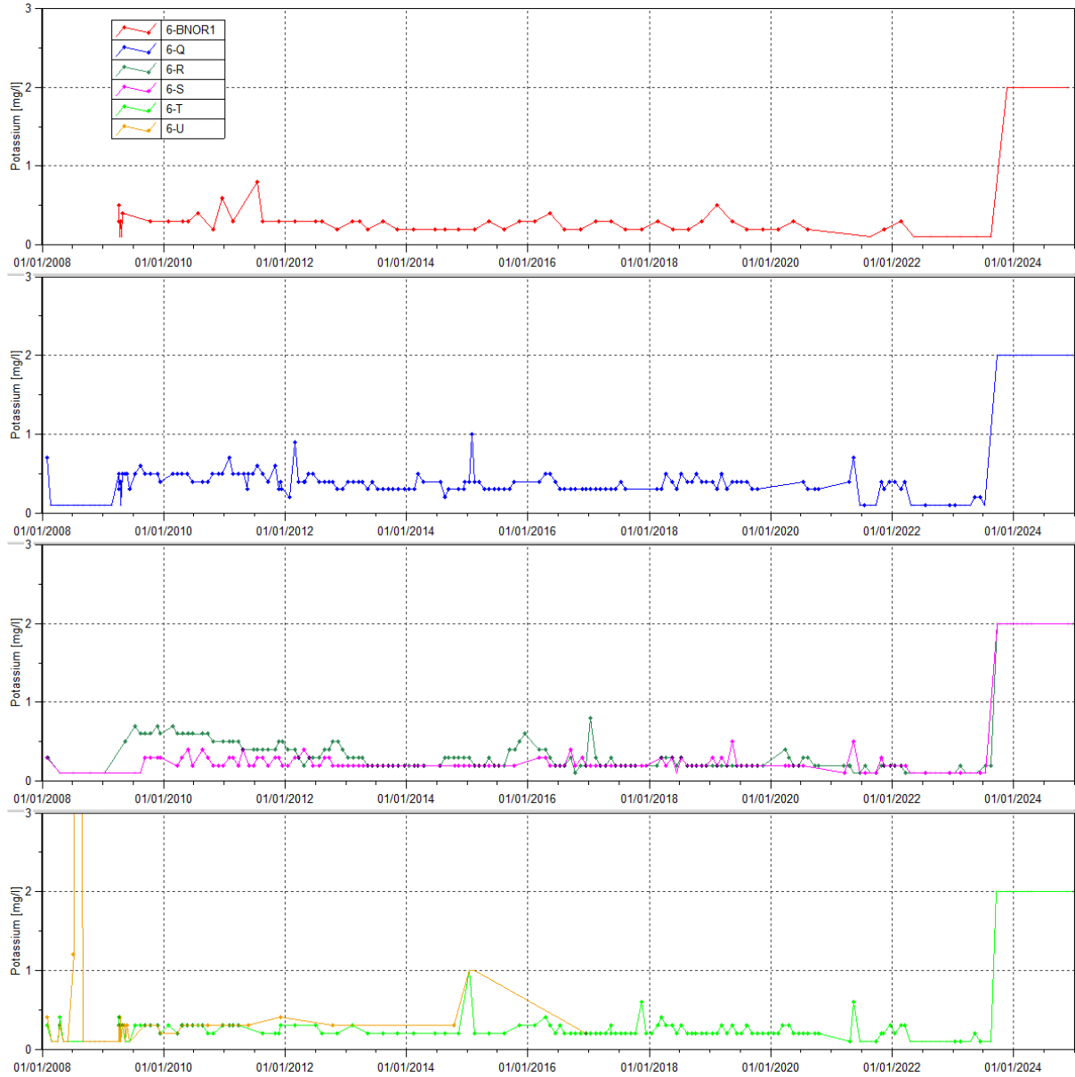
Figure 22 : Concentrations en potassium pour les stations 6-BNOR1, 6-Q, 6-R, 6-S, 6-T et 6-U entre janvier 2008 et le 1er janvier 2025
