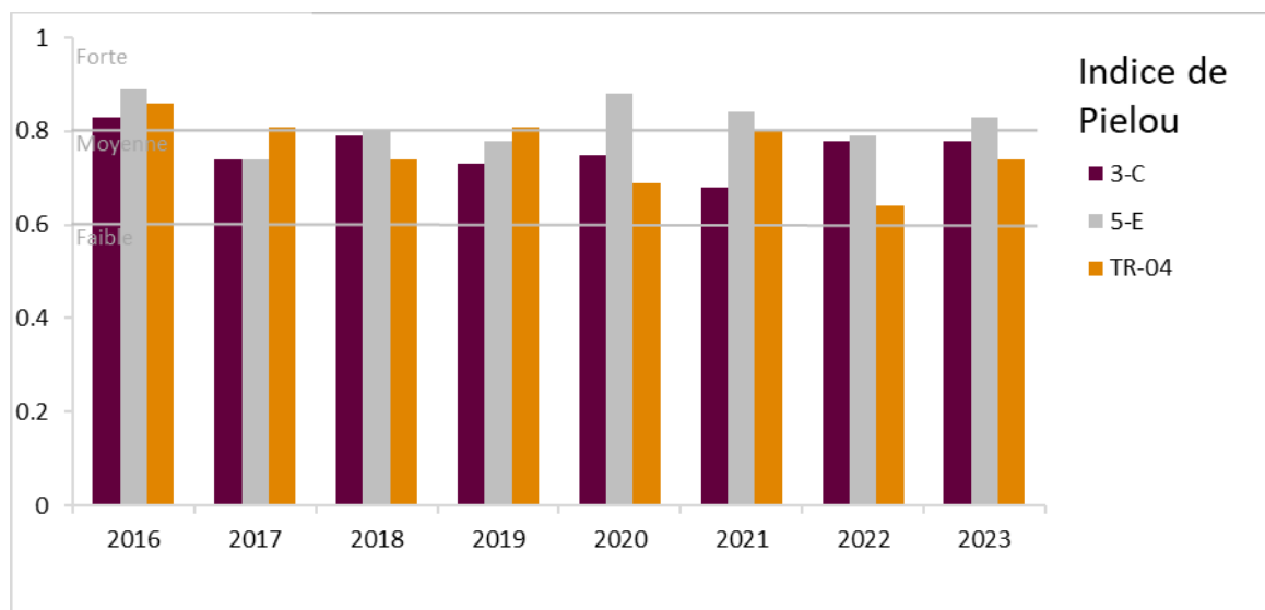
Figure 116 : Indices de Pielou des stations 3-C, 5-E et TR-04
