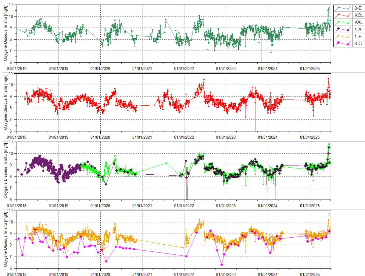
Figure 38 : Oxygène dissous des stations 3-E, KOL, 1-A, KAL, 1-E et 3-C entre janvier 2018 et le 1er juillet 2025
