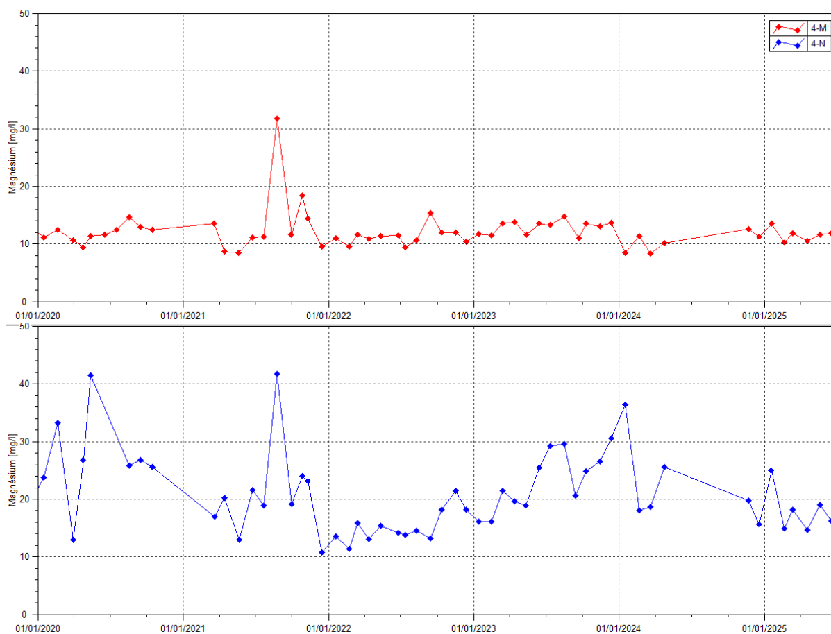
Figure 64 : Données de magnésium des stations 4-M et 4-N entre janvier 2020 et le 1er juillet 2025
