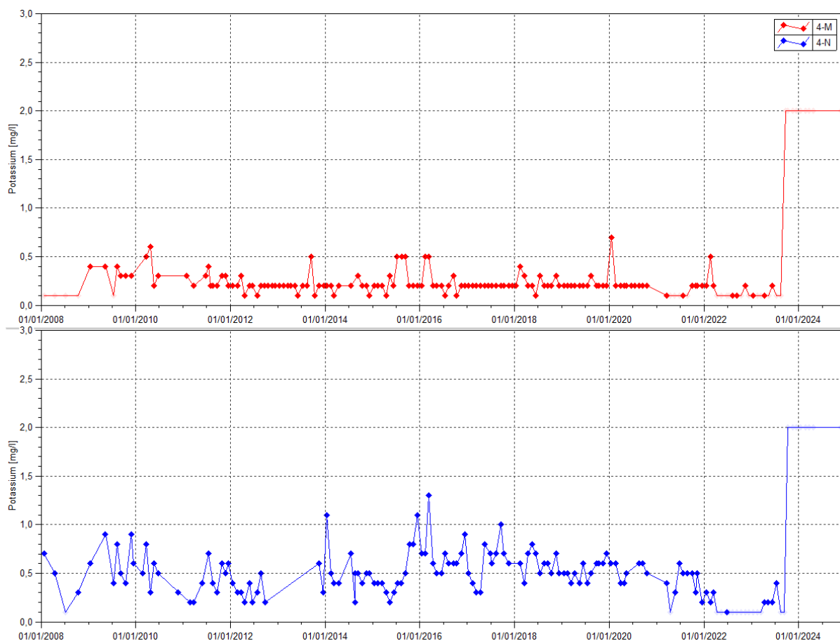
Figure 59 : Données de potassium des stations 4-M et 4-N entre janvier 2008 et le 1er juillet 2025
