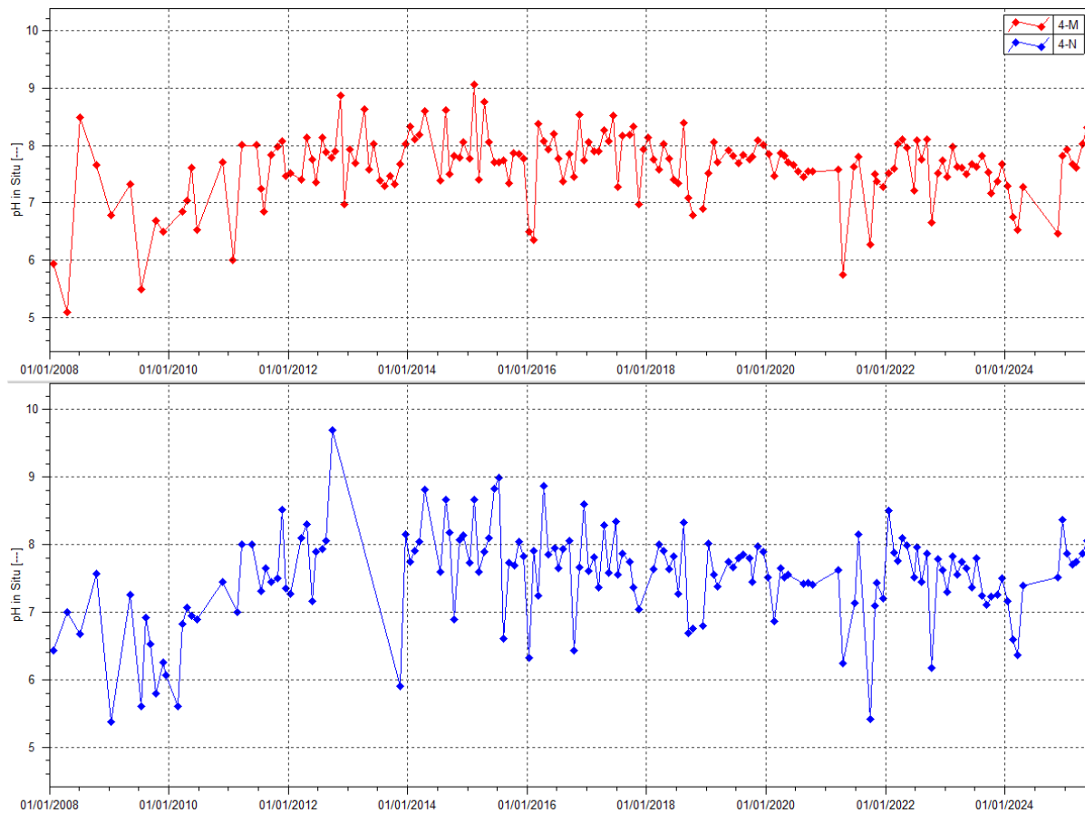
Figure 36 : Données de pH des stations 4-M et 4-N entre janvier 2008 et le 1er juillet 2025
