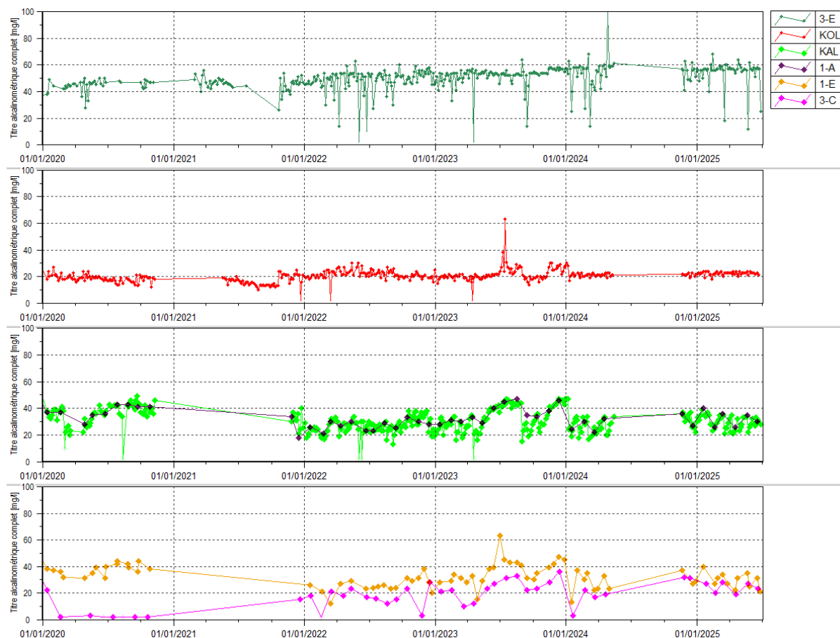
Figure 40 : Alcalinité des stations 3-E, KOL, 1-A, 1-E et 3-C entre janvier 2020 et le 1er juillet 2025
