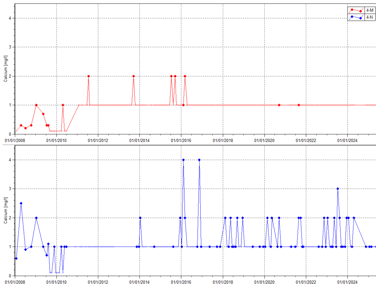
Figure 55 : Données de calcium des stations 4-M et 4-N entre janvier 2008 et juillet 2025
