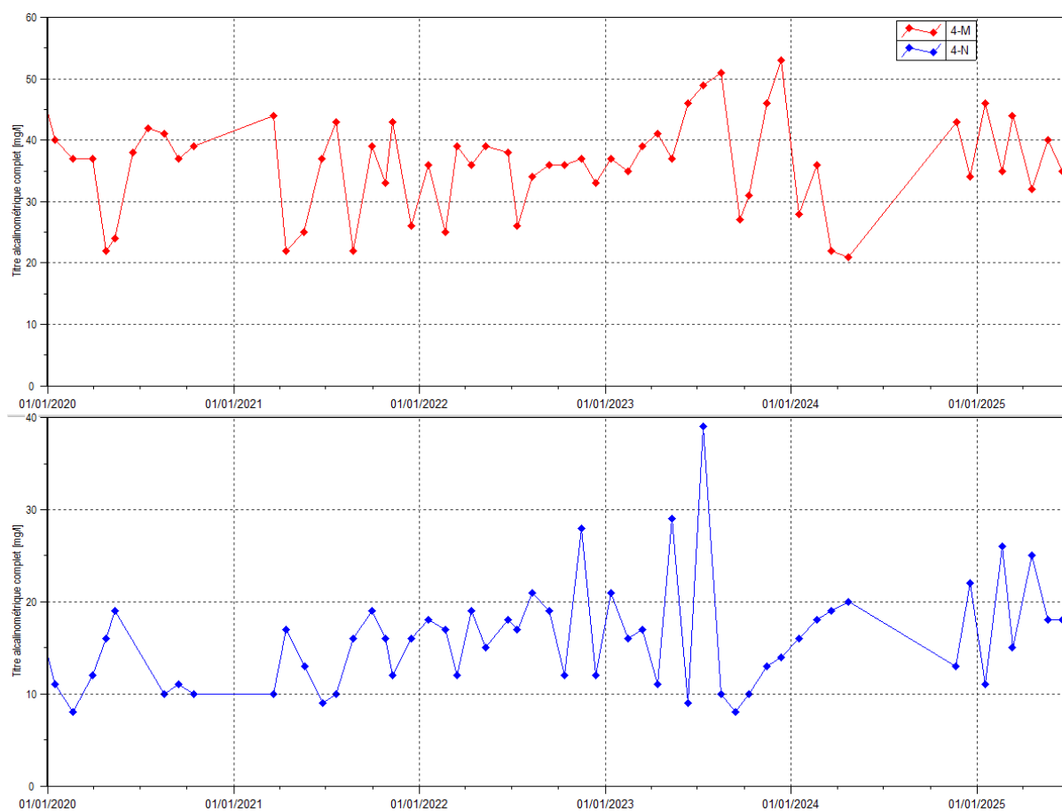
Figure 42 : Alcalinité des stations 4-M et 4-N entre janvier 2020 et le 1er juillet 2025
