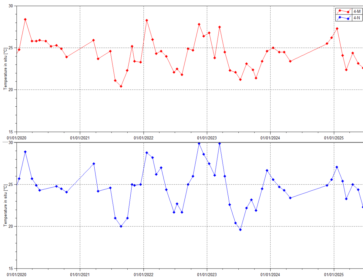
Figure 33 : Données de températures mensuelles aux stations 4-M et 4-N entre janvier 2020 et le 1er juillet 2025
