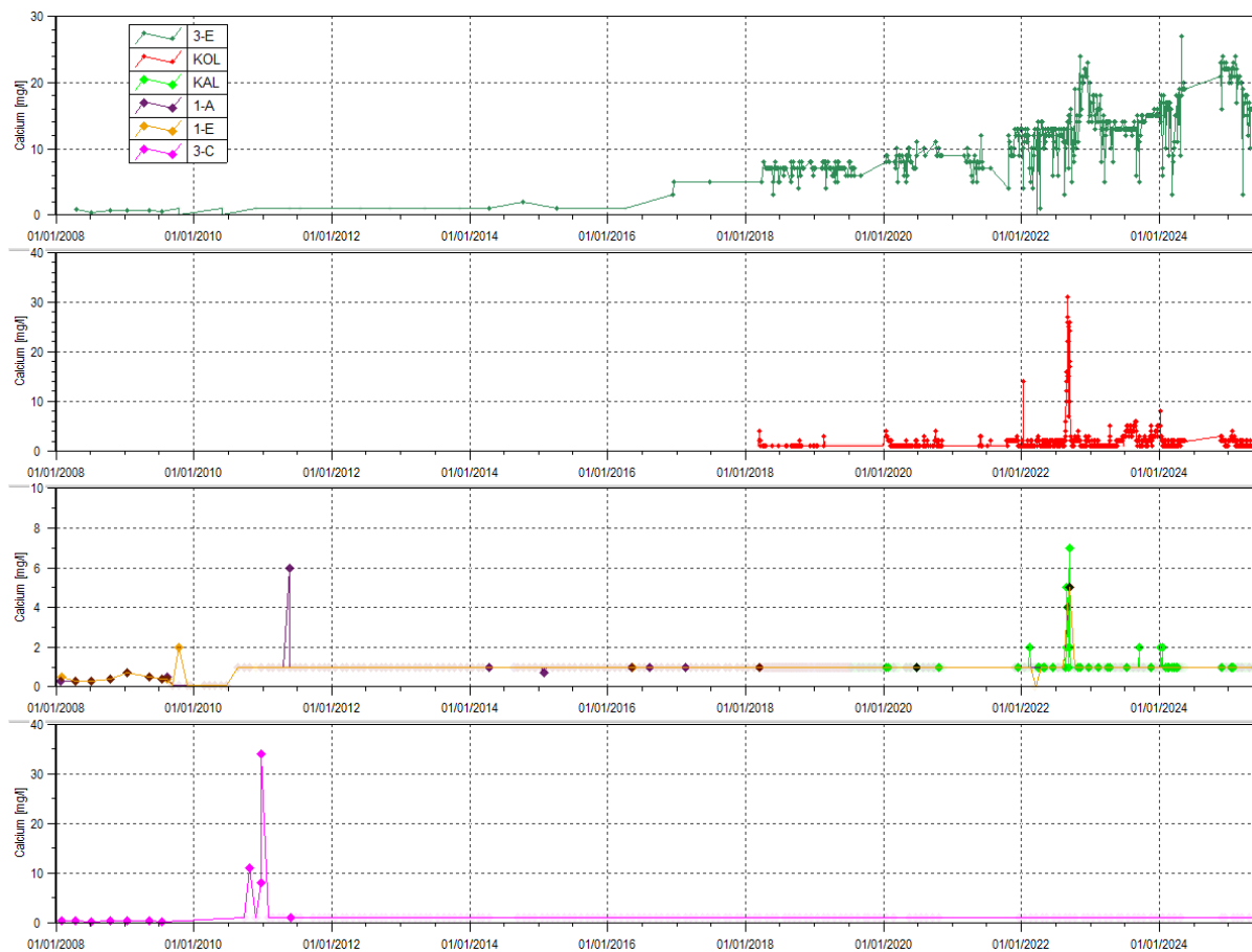
Figure 53 : Calcium des stations 3-E, KOL, KAL, 1-A, 1-E et 3-C depuis 2008
