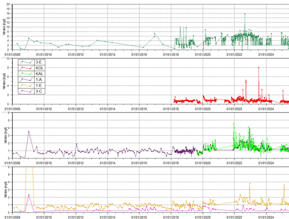
Figure 47 : Nitrates des stations 3-E, KOL, 1-A, KAL, 1-E et 3-C entre janvier 2008 et le 1er juillet 2025
