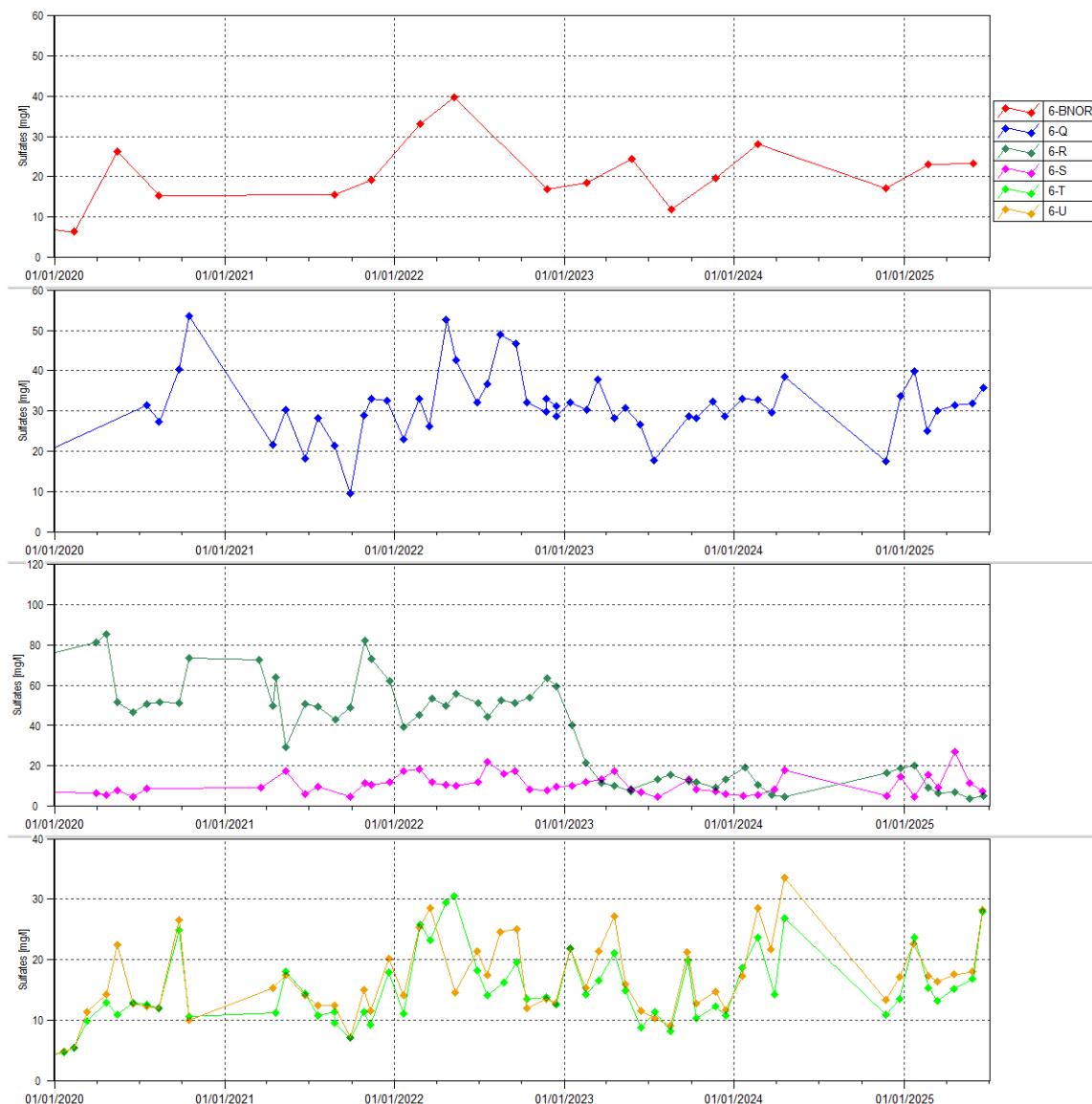
Figure 11 : Concentration en sulfates pour les stations 6-BNOR1, 6-Q, 6-R, 6-S, 6-T et 6-U entre janvier 2020 et le 1 er juillet 2025
