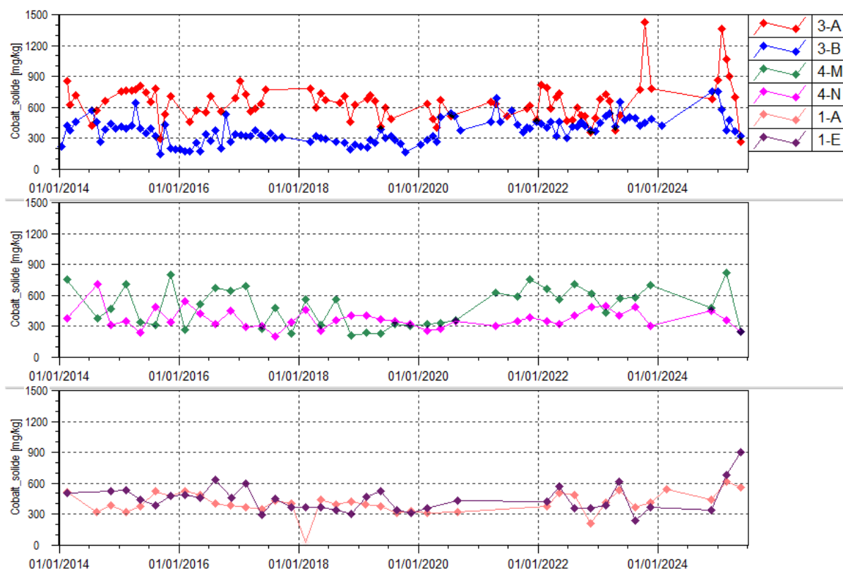
Figure 95 : Concentration en cobalt dans les sédiments des stations de la Kwé entre janvier 2014 et juillet 2025
