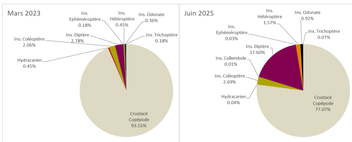
Figure 120 : Composition du peuplement de macro-invertébrés benthiques, DOL-10 mars 2023 et juin 2025
