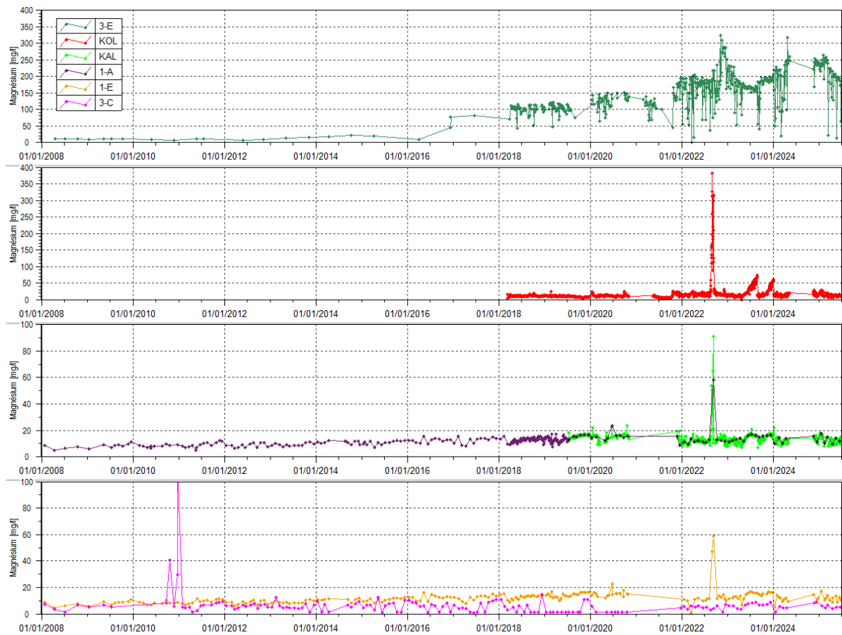
Figure 61 : Magnésium des stations 3-E, KOL, KAL, 1-A, 1-E et 3-C depuis 2008
