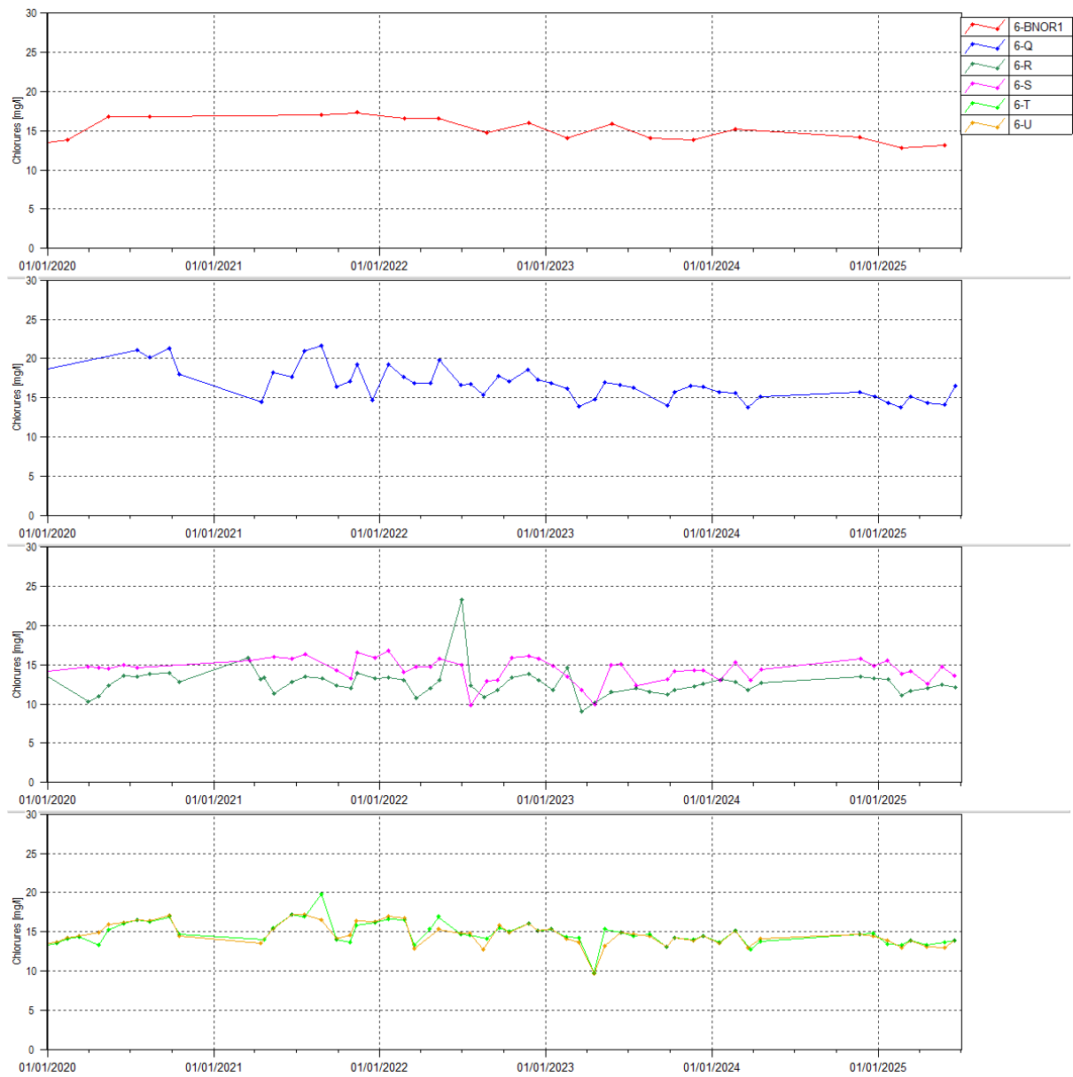
Figure 13 : Concentration en chlorures pour les stations 6-BNOR1, 6-Q, 6-R, 6-S, 6-T et 6-U entre janvier 2020 et le 1 er juillet 2025
