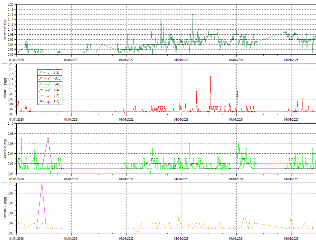
Figure 70 : Chrome VI des stations 3-E, KOL, KAL, 1-A, 1-E et 3-C entre janvier 2020 et le 1er juillet 2025
