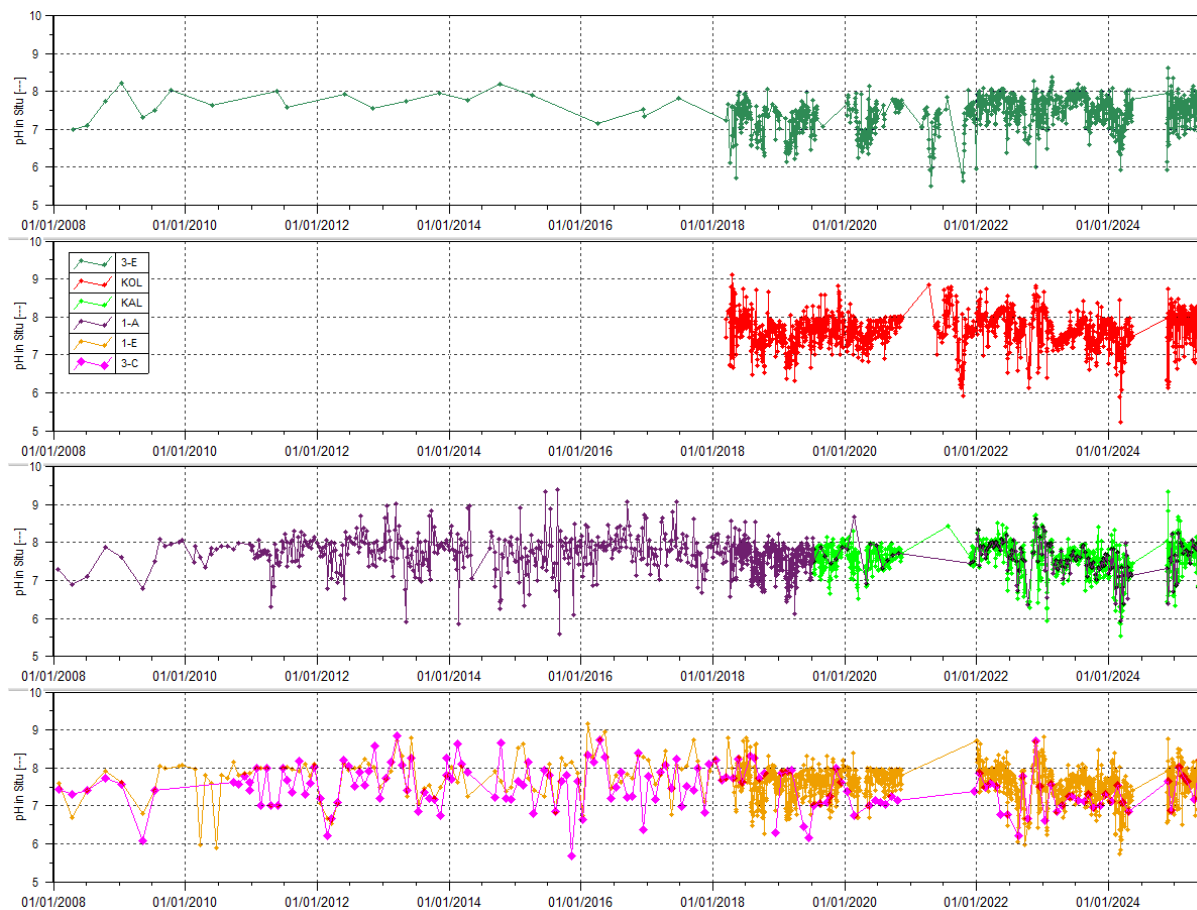
Figure 34 : Mesures de pH aux stations 3-E, KOL, KAL, 1-A, 1-E et 3-C entre janvier 2008 et le 1er juillet 2025
