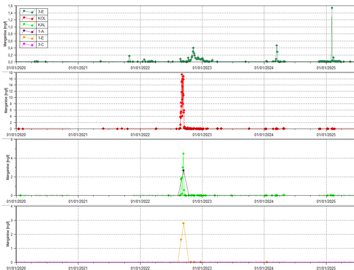
Figure 74 : Données de manganèse des stations 3-E, KOL, KAL, 1-A, 1-E et 3-C de janvier 2020 à juillet 2025
