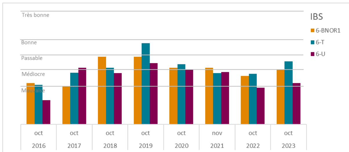
Figure 105 : Résultats IBS (version 2016) des stations 6-bnor1, 6-T et 6-U du creek de la Baie Nord
