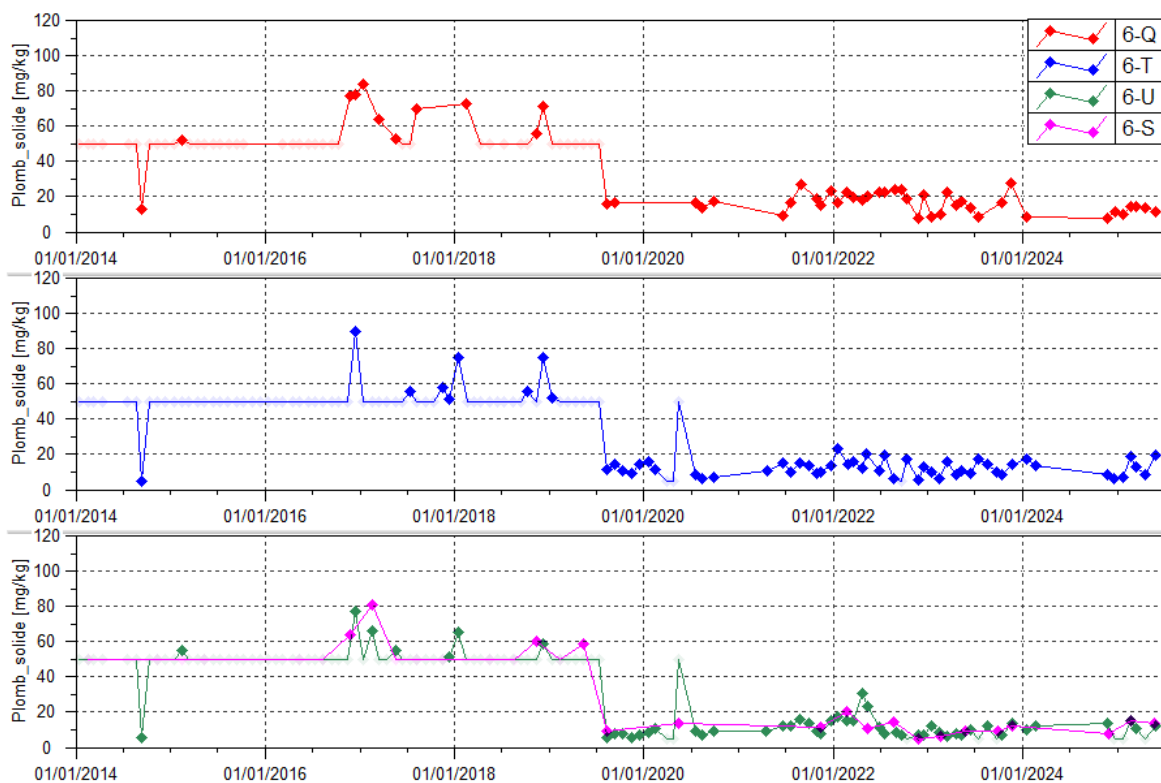
Figure 93 : Concentration en plomb dans les sédiments des stations du creek de la Baie Nord entre janvier 2014 et juillet 2025
