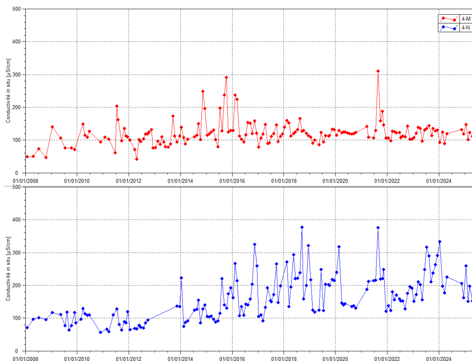
Figure 29 : Données de conductivité aux stations 4-M et 4-N entre janvier 2008 et le 1er juillet 2025
