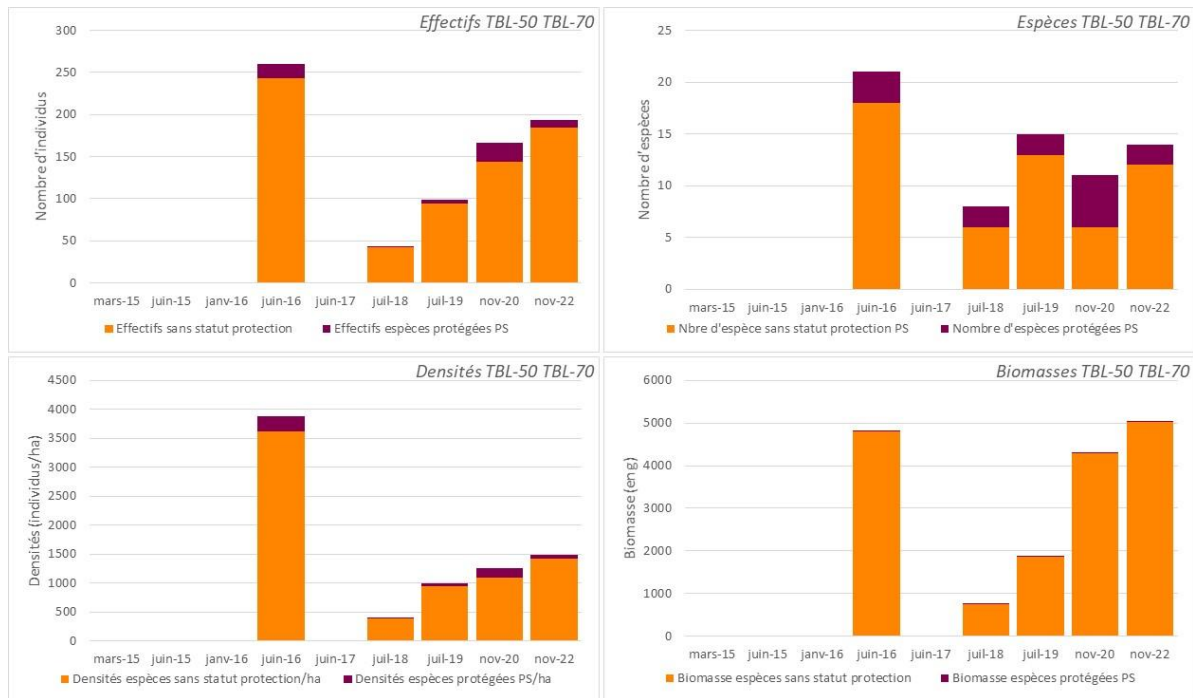
Figure 129 : Evolution des descripteurs biologiques de la faune aquatique au niveau de la rivière Trou Bleu entre juin 2016 et novembre 2022 (effectif, espèces, biomasses et densités)
