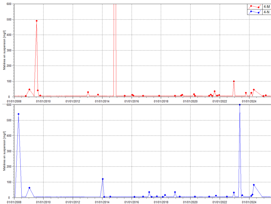
Figure 85 : Données de MES des stations 4-M et 4-N entre janvier 2008 et le 1er juillet 2025
