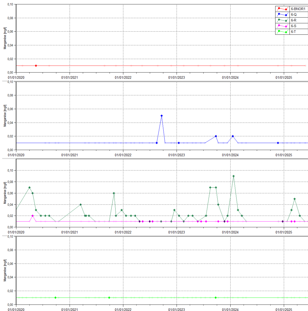
Figure 15 : Concentration en manganèse pour les stations 6-BNOR1, 6-Q, 6-R, 6-S et 6-T entre janvier 2020 et le 1 er juillet 2025
