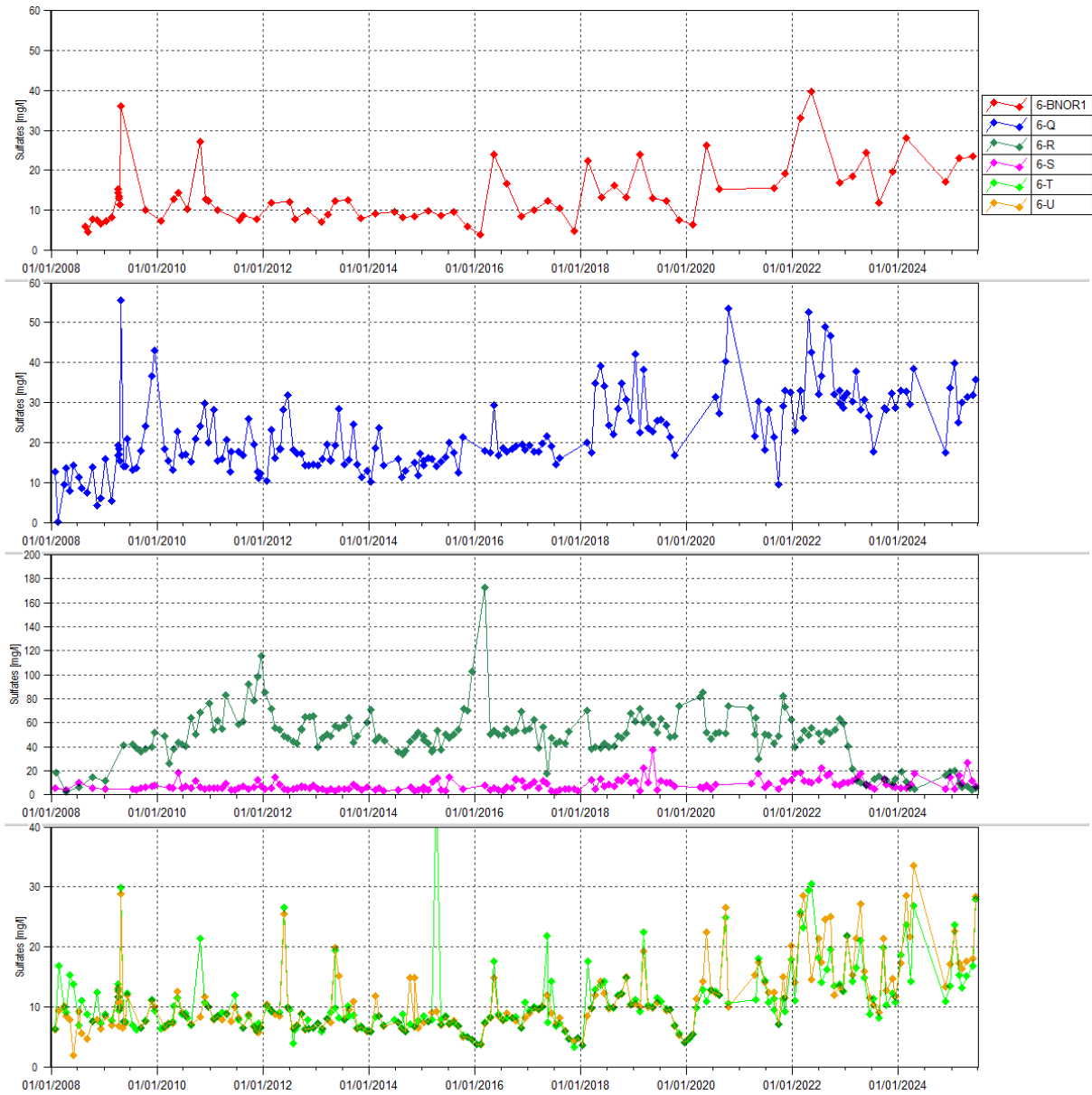
Figure 10 : Concentration en sulfates pour les stations 6-BNOR1, 6-Q, 6-R, 6-S, 6-T et 6-U entre janvier 2008 et le 1 er juillet 2025
