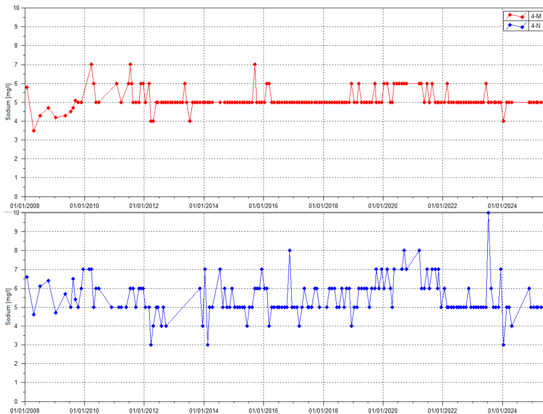
Figure 67 : Données de sodium des stations 4-M et 4-N entre janvier 2008 et le 1er juillet 2025
