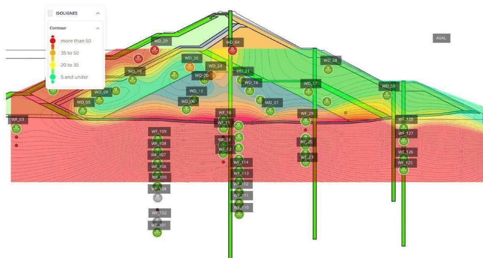
Figure 9 : Isoligne de pression interstitielle en kPa – Chainage 500 en date du 31/12/2025
