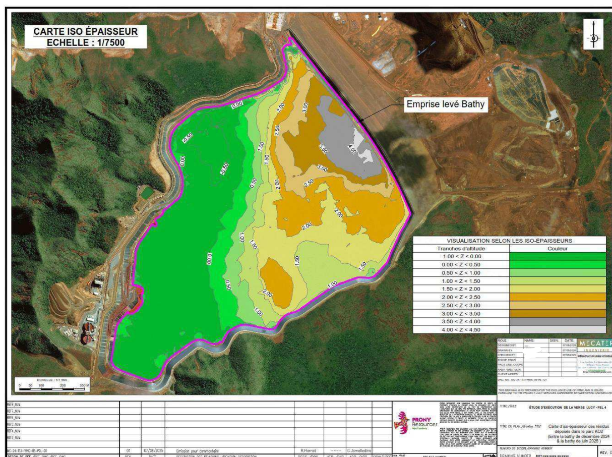
Figure 3 : Plan de dépôt des résidus entre décembre 2024 et juin 2025 - Carte d'iso-épaisseur des résidus déposés pendant cette période
