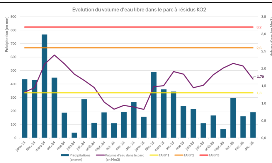
Figure 6 : Variation du volume d'eau par rapport aux valeurs seuils du TARP
