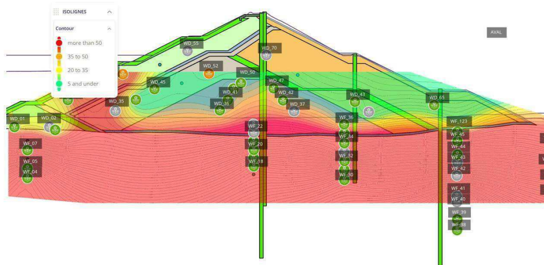
Figure 10 : Isoligne de pression interstitielle en kPa – Chainage 700 en date du 31/12//2025
