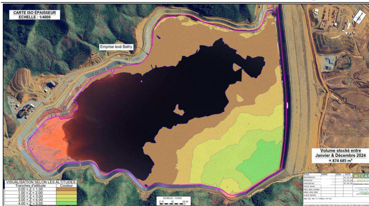
Figure 2 : Plan de dépôt des résidus entre janvier et décembre 2024 – Carte d'iso-épaisseur de résidus déposés pendant cette période
