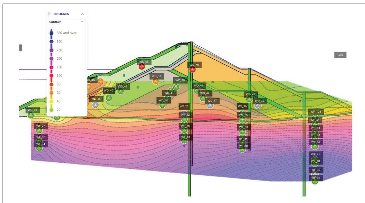
Figure 11 : Isoligne de pression interstitielle en kPa - Chainage 700 en date du 31/03/2026
