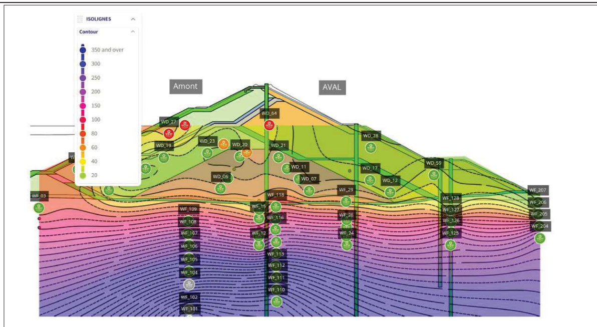
Figure 10 : Isoligne de pression interstitielle en kPa - Chainage 500 en date du 31/03/2026
