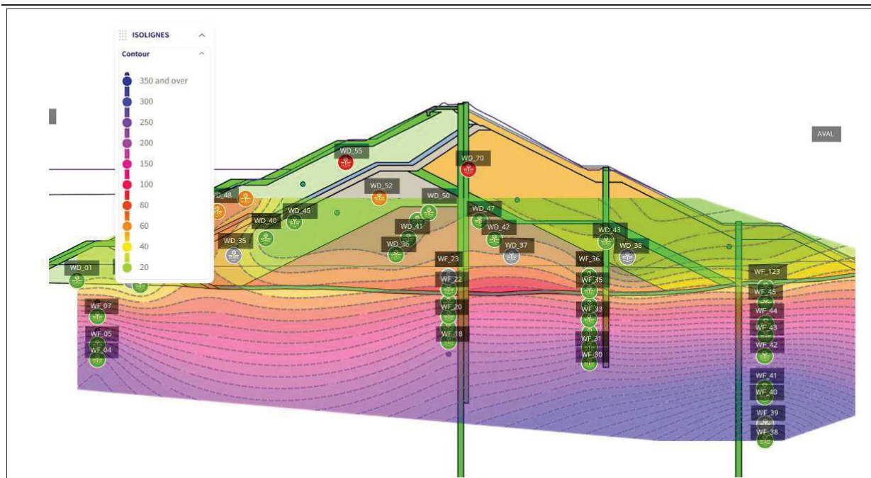
Figure 7 : Isoligne de pression interstitielle en kPa – Chainage 700 au 30/04/2026
