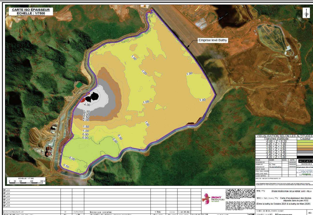
Figure 2 : Plan de déposition des résidus entre octobre 2025 et mars 2026 - Carte d'iso-épaisseur des résidus déposés pendant cette période
