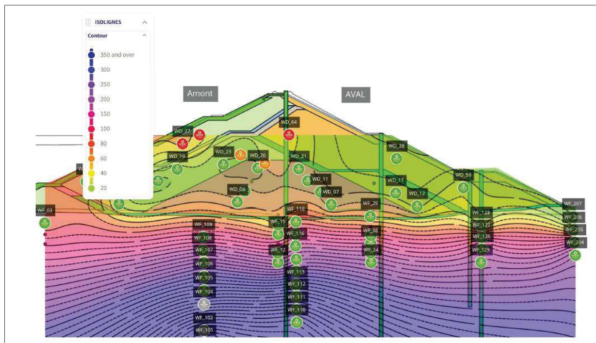
Figure 6 : Isoligne de pression interstitielle en kPa – Chainage 500 au 30/04/2026
