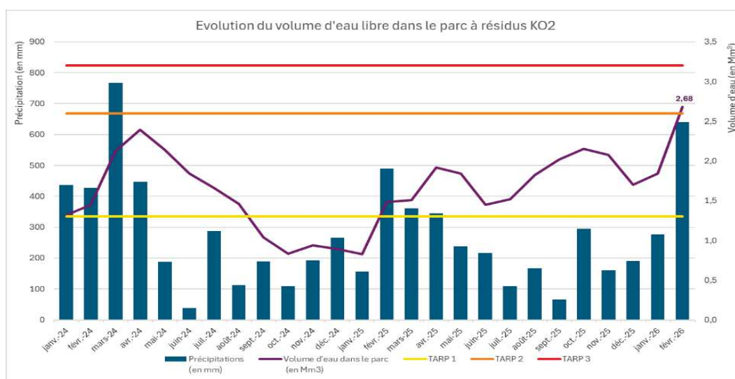
Figure 2 : Variation du volume d'eau par rapport aux valeurs seuils du TARP
