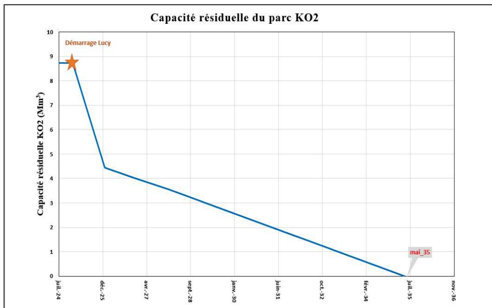
Figure 4 : Graphique - capacité résiduelle dans KO2 avec projet Lucy
