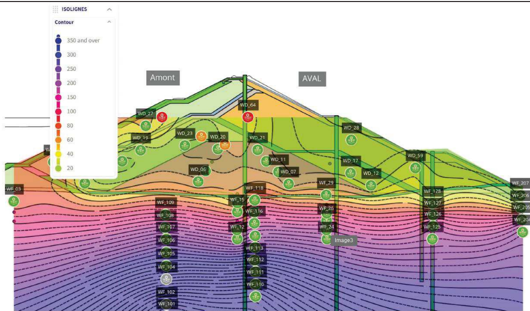
Figure 9 : Isoligne de pression interstitielle en kPa – Chainage 500 en date du 28/02/2026
