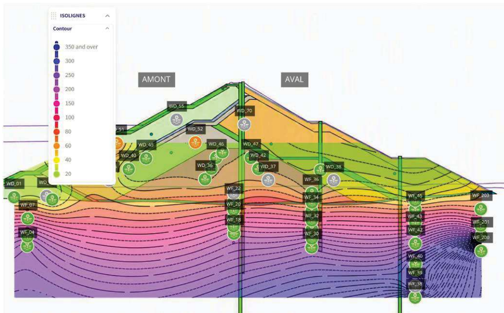
Figure 10 : Isoligne de pression interstitielle en kPa – Chainage 700 en date du 28/02/2026
