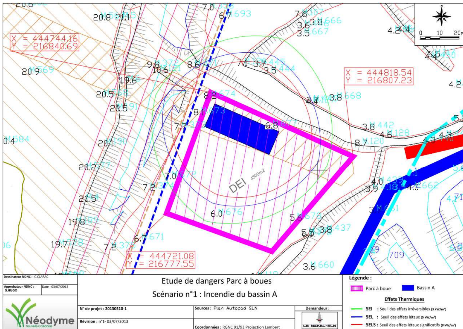
Figure 4 : cartographie de la modélisation du scénario d'incendie du bassin A
