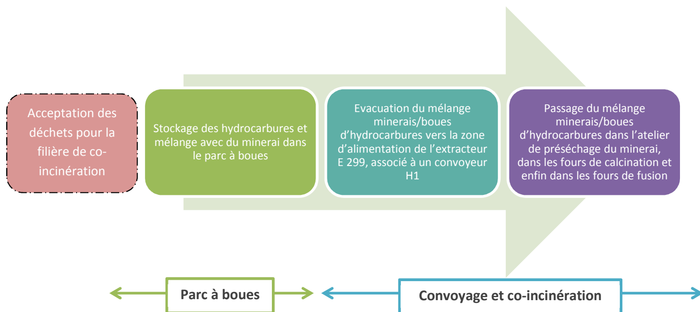
Figure 1 : étapes de co-incinération des boues d'hydrocarbures
