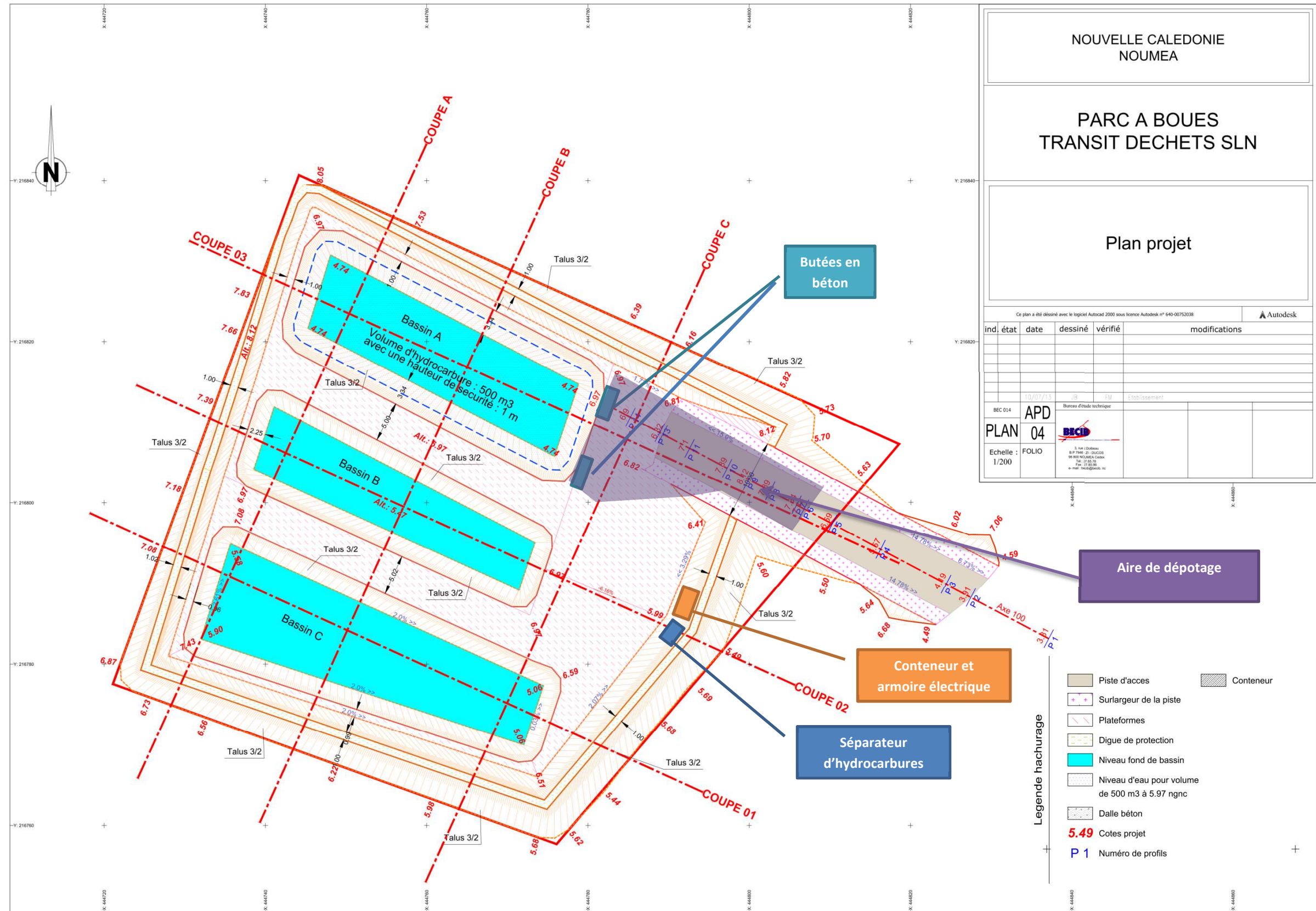
Figure 13 : schéma général du futur parc à boues
