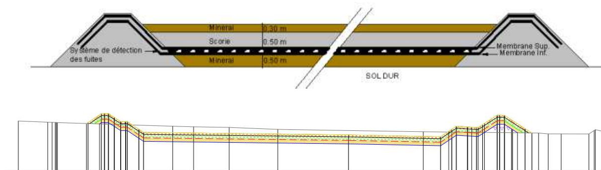
Figure 12: Schéma en coupe du futur parc à boues
