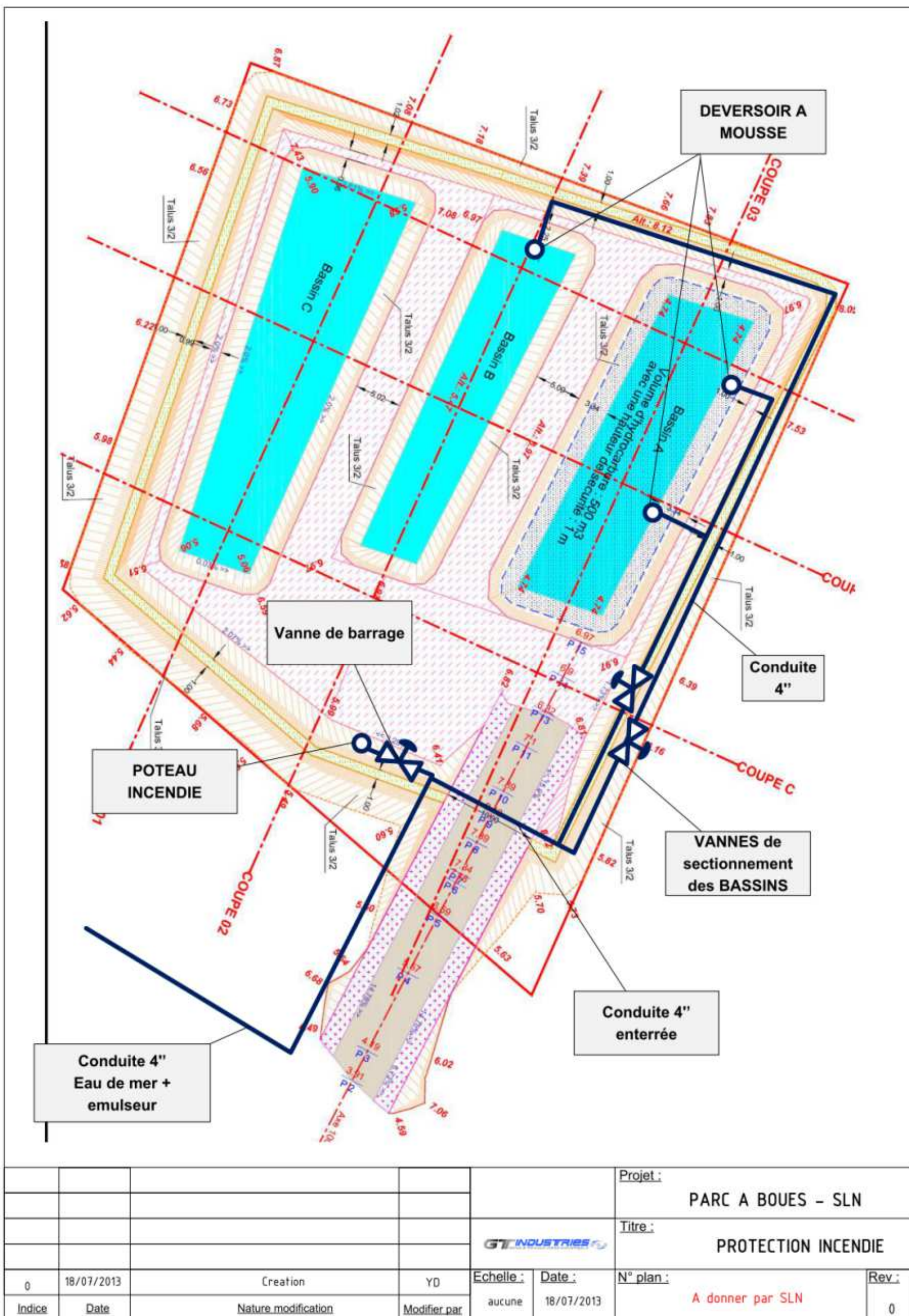
Figure 14 : schéma de la protection incendie prévue pour le parc à boues
