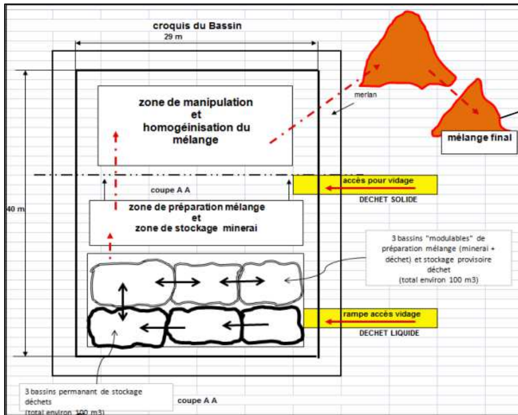
Figure 4 : Schéma de principe du parc à boues actuel
