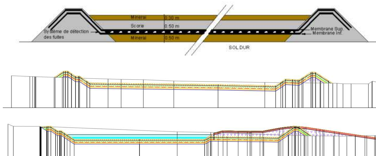
Figure 12: Schémas en coupe du futur parc à boues
