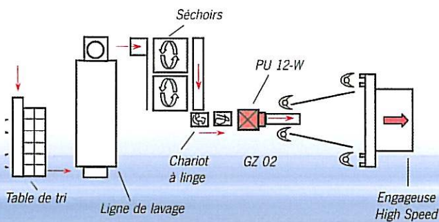
Tri du linge sale avec intégration du PU 12-W en amont de l'engageuse High Speed
