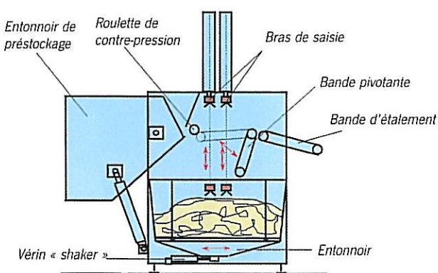
Tri du linge propre avec intégration du PU 12-D en amont de l'Ergomat Automatique
