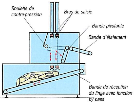
Tri du linge propre avec intégration du PU 12-U en amont de la ligne combinée
