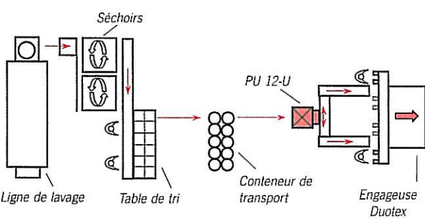
Tri du linge propre avec intégration du PU 12-U en amont de la ligne combinée
