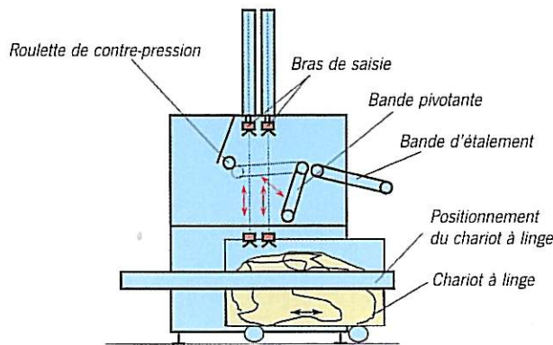
Tri du linge sale avec intégration du PU 12-W en amont de l'engageuse High Speed
