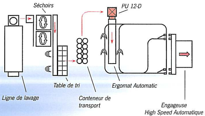
Tri du linge propre avec intégration du PU 12-D en amont de l'Ergomat Automatique
