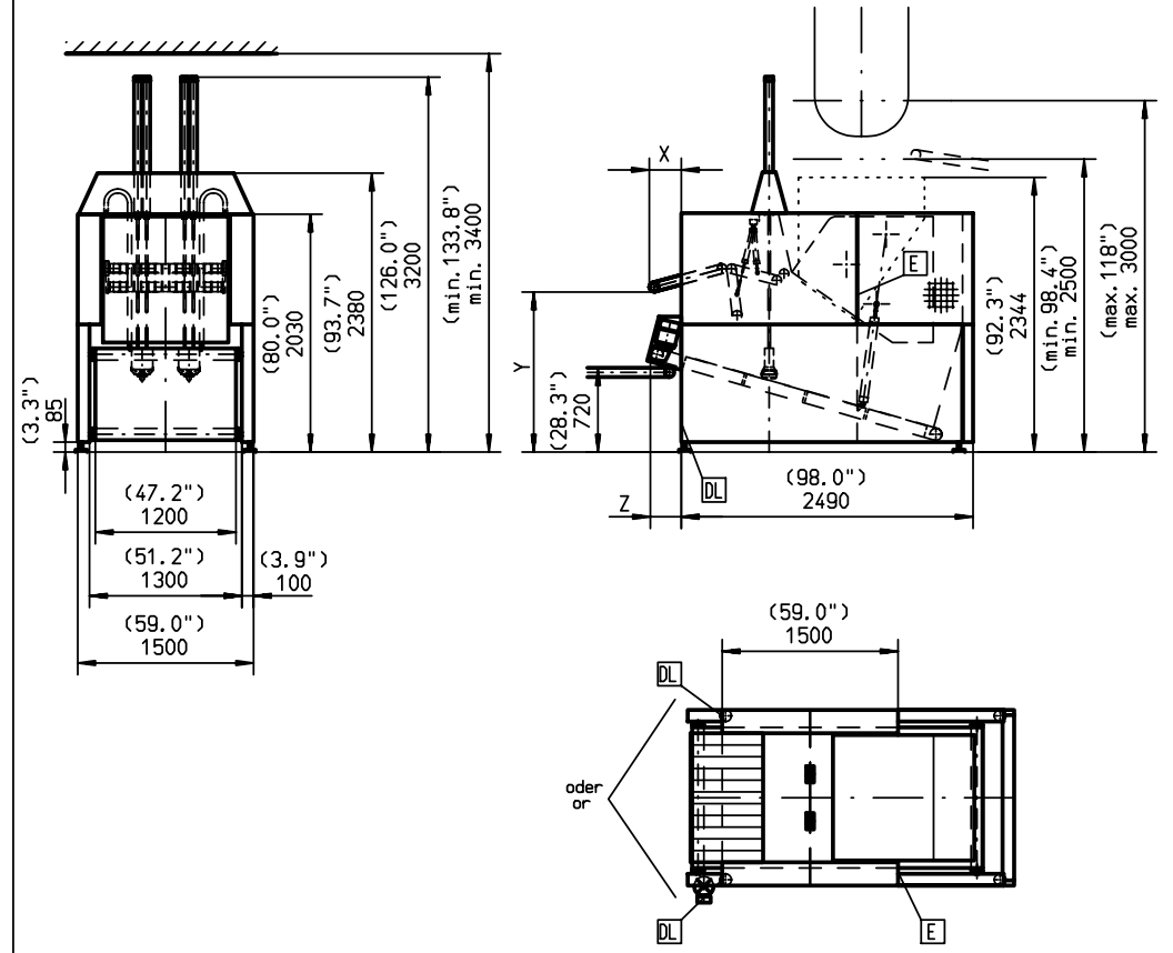
mit Trichter und Speicherband with funnel and storage belt conveyor
