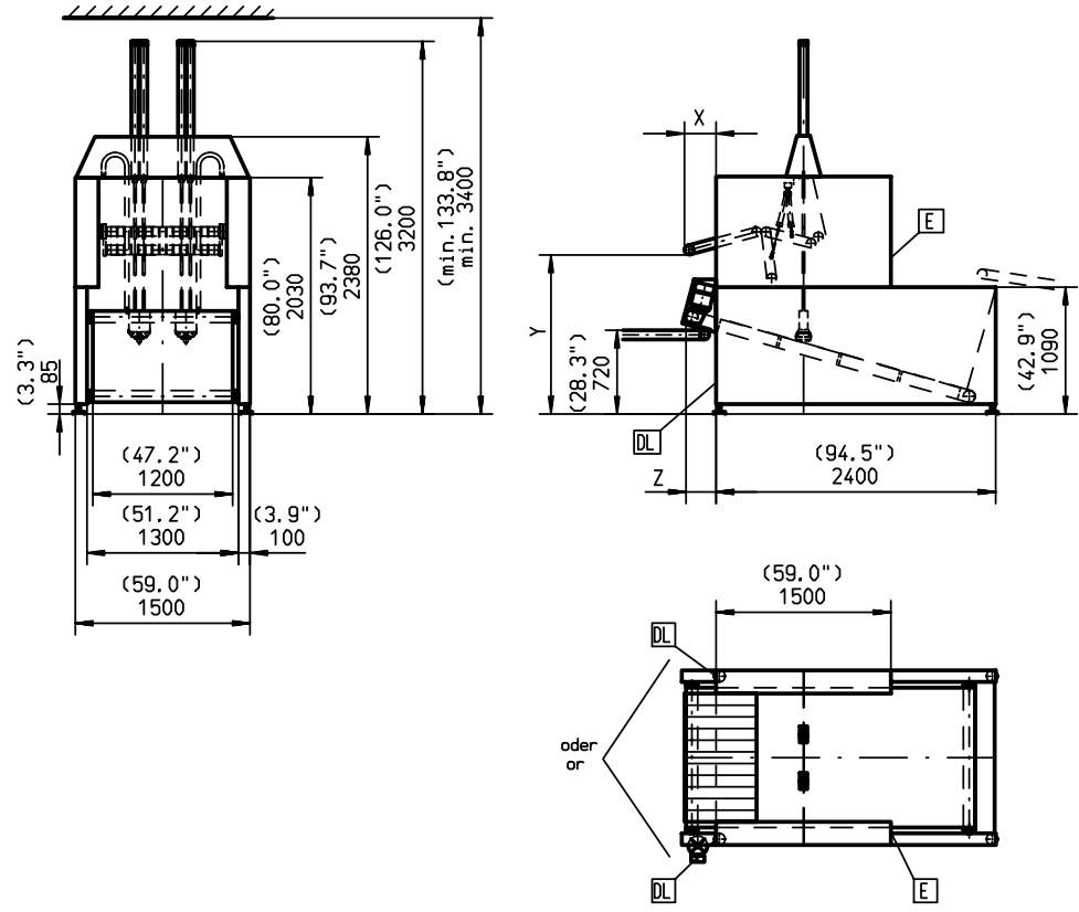
mit Speicherband with storage belt conveyor
