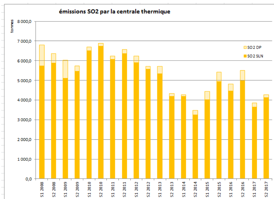
Emissions de SO2 de la centrale thermique avec part SLN et Distribution Publique (DP)
