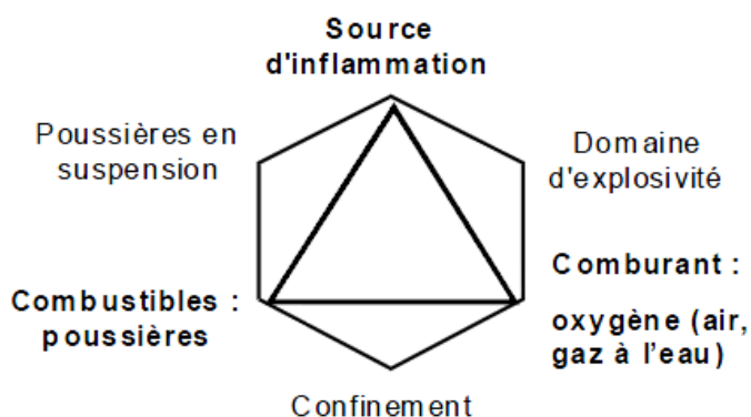
Figure 56 : Hexagone de l'explosion
