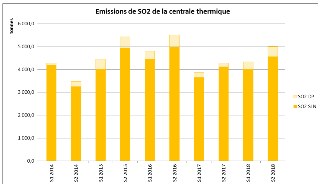
Emissions de SO2 de la centrale thermique avec part SLN et Distribution Publique (DP)
