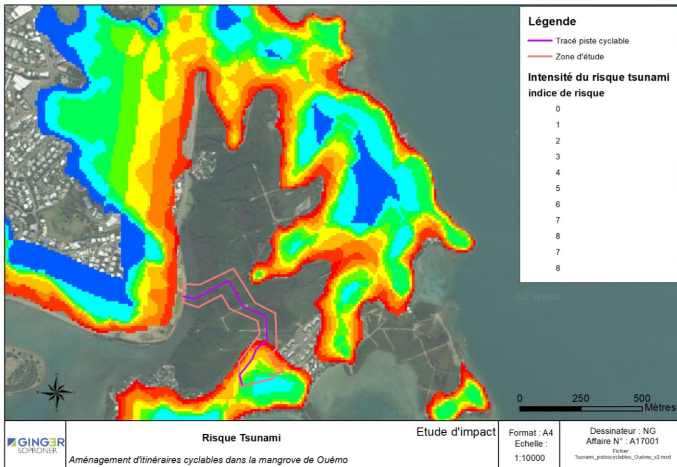
Figure 60 : Risque Tsunami
