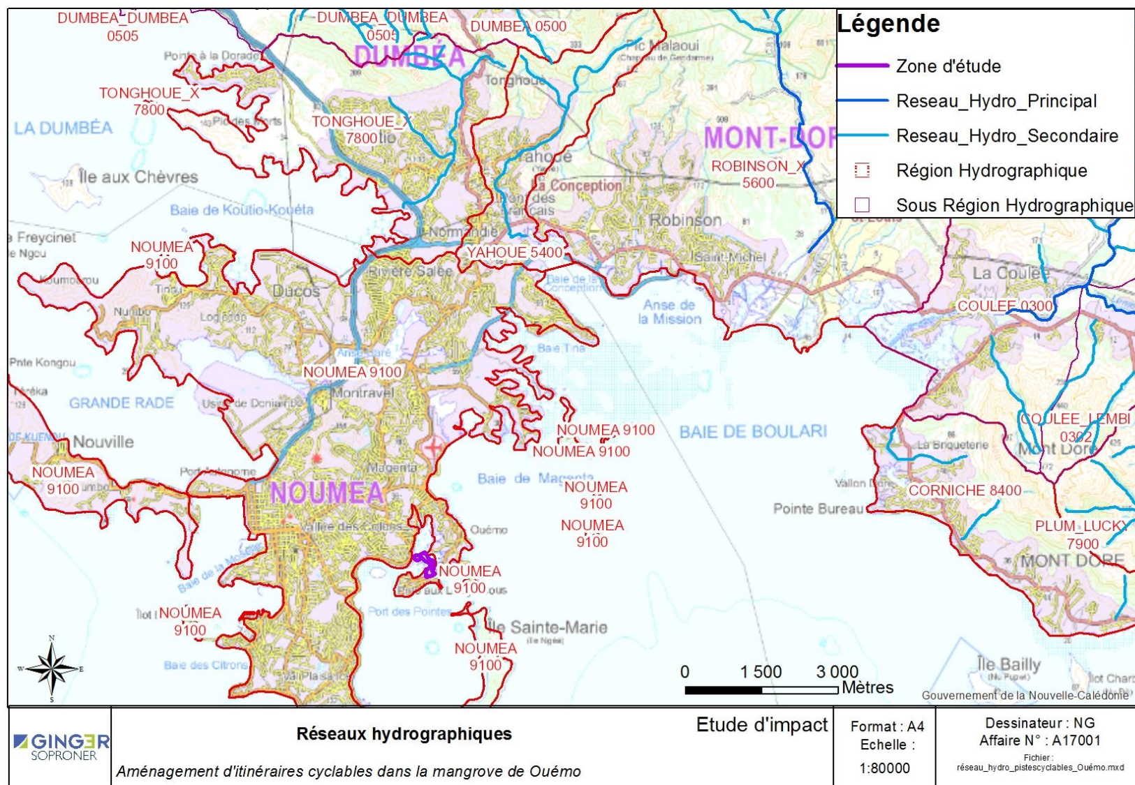
Figure 32 : Réseaux hydrographiques
