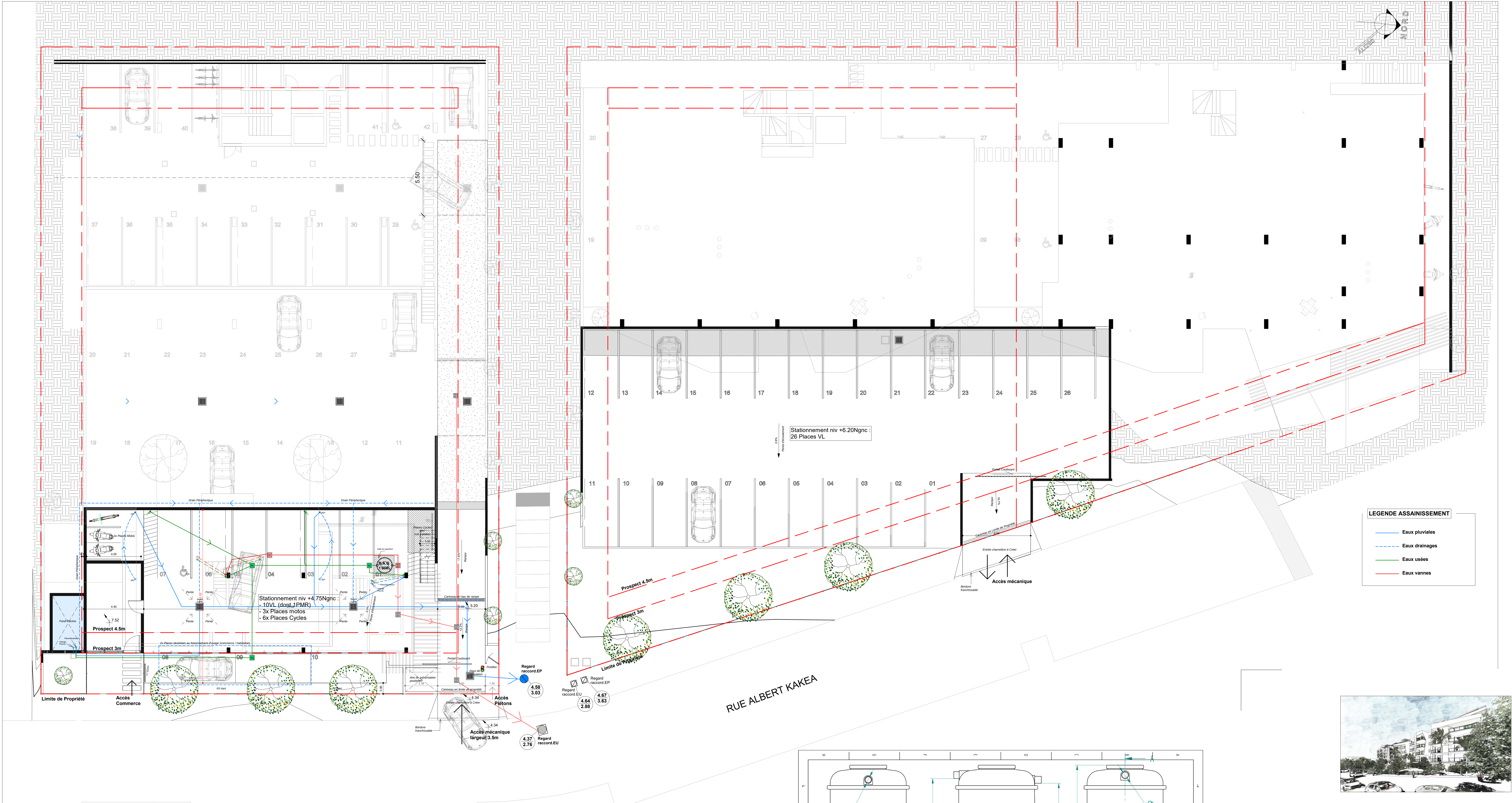
SCHEMA ASSAINISSEMENT Niv. +4.75ngnc Ech:1/100
