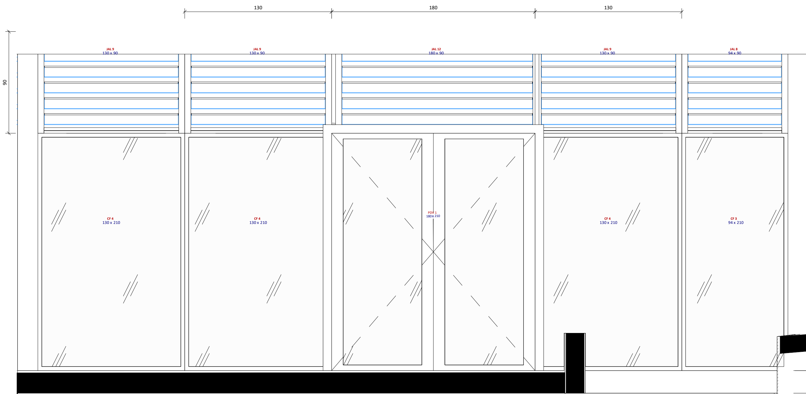
Assemblage 2 1 : 20
